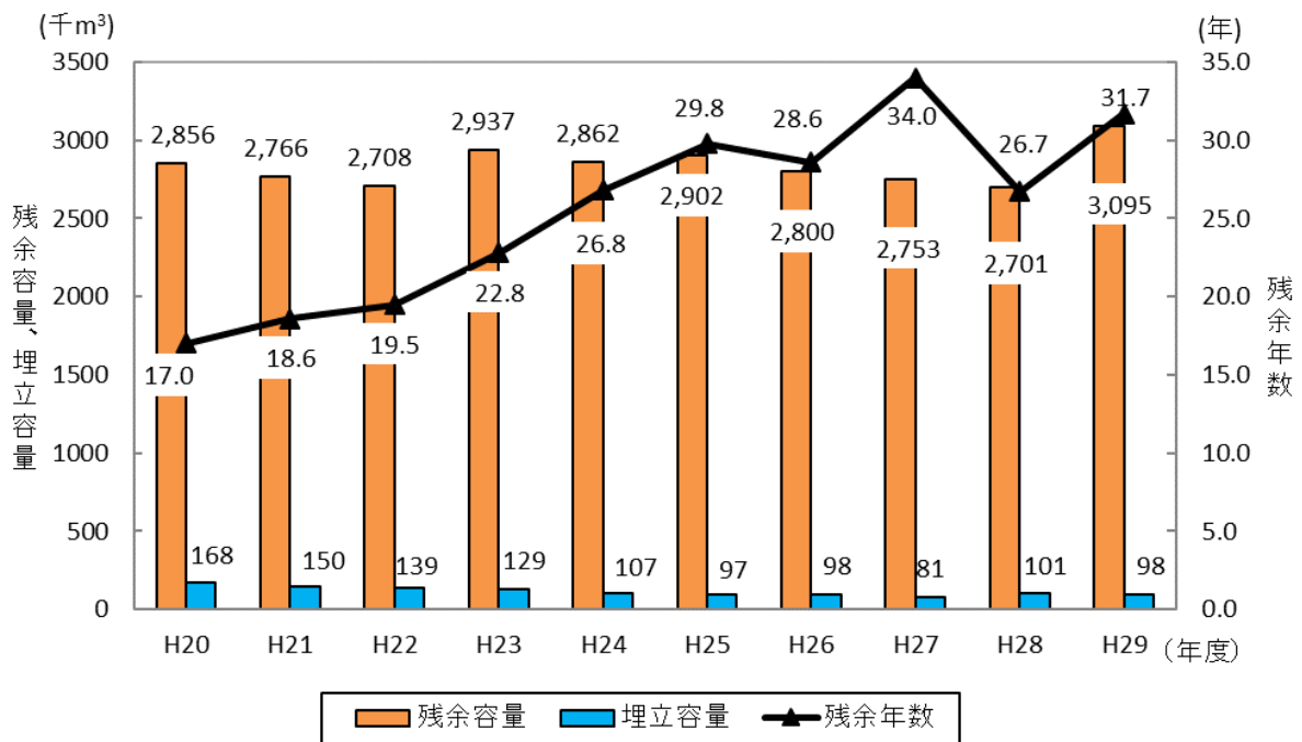
図 9 最終処分場の残余容量、最終処分量、残余年数の経年変化
