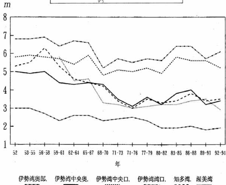
図 - 2 - 2 伊勢湾・三河湾における透明度の推移（上図は調査位置） 資料）石田基雄・原保・伊勢・三河湾における水質変動と富栄養化について （1996年、愛知県水産試験場研究報告第3号）
