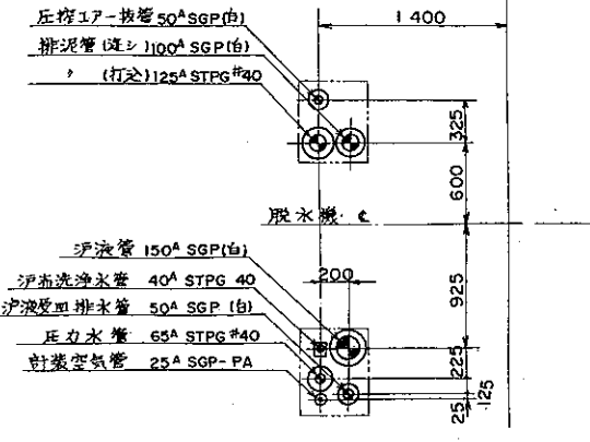
脱水機開口部詳細 S=1:30
