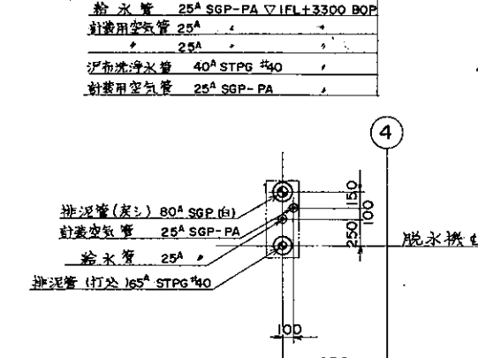
脱水機出口部詳細
