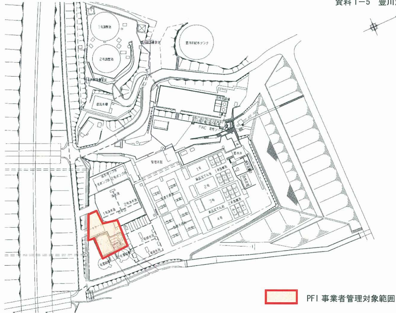
資料 1-5 豊川浄水場平面図
