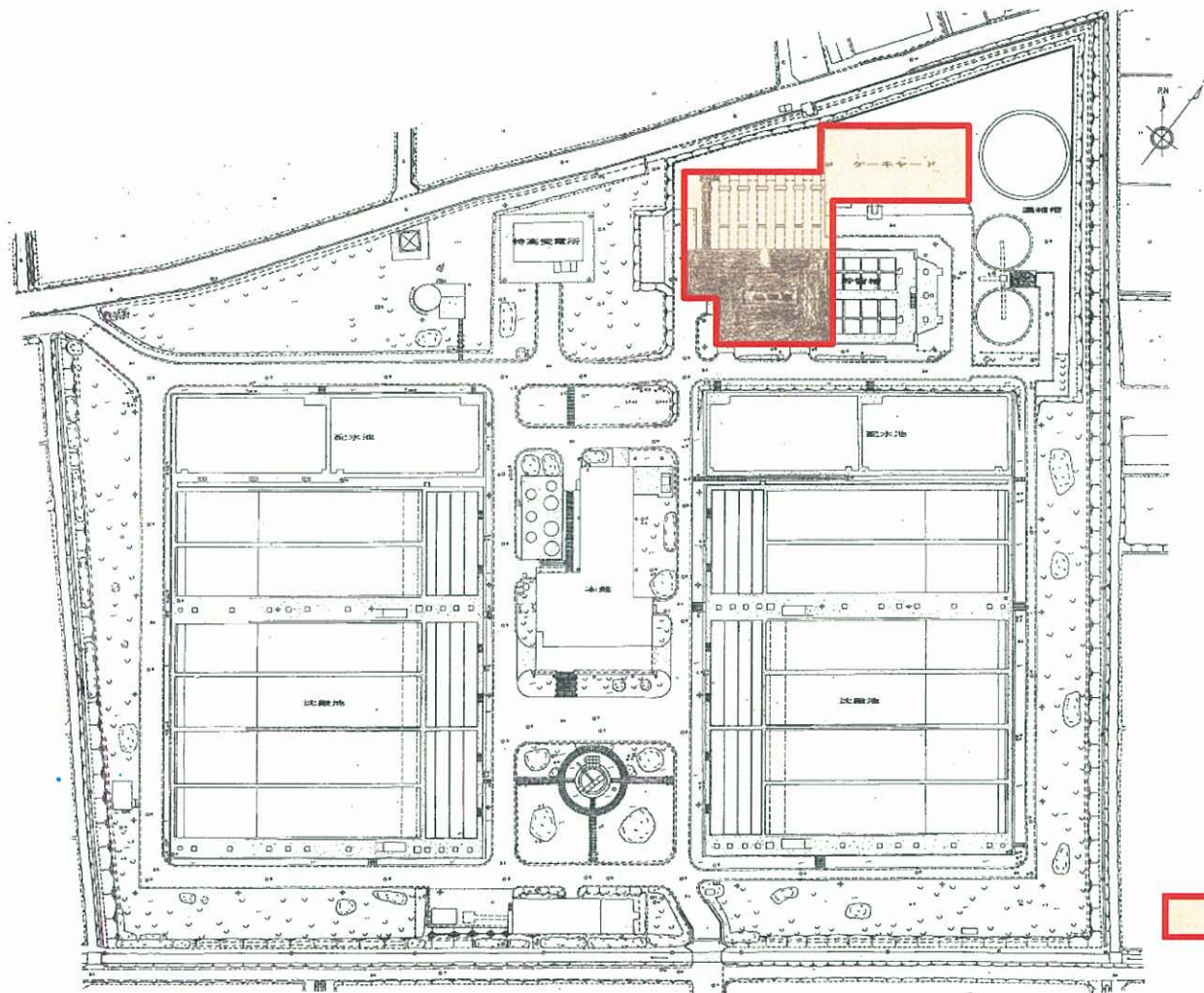
資料 1-3 安城浄水場平面図
