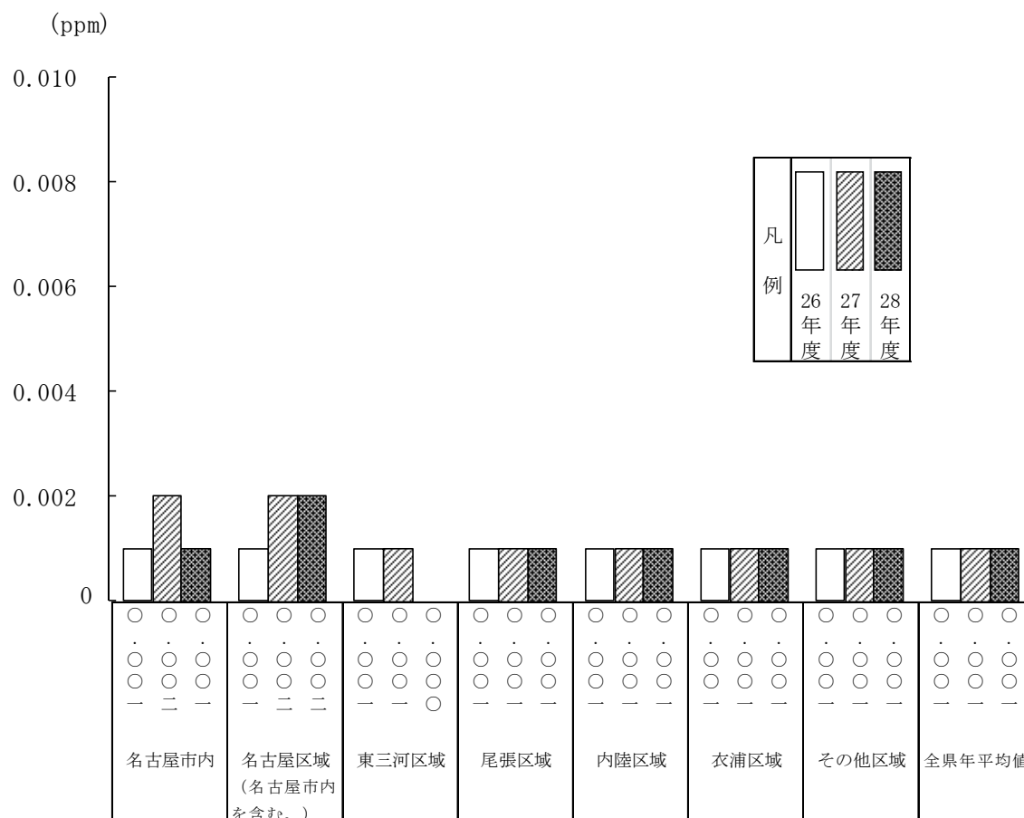
図1-4 二酸化硫黄の区域別年平均値の経年変化 (一般環境大気測定局)
