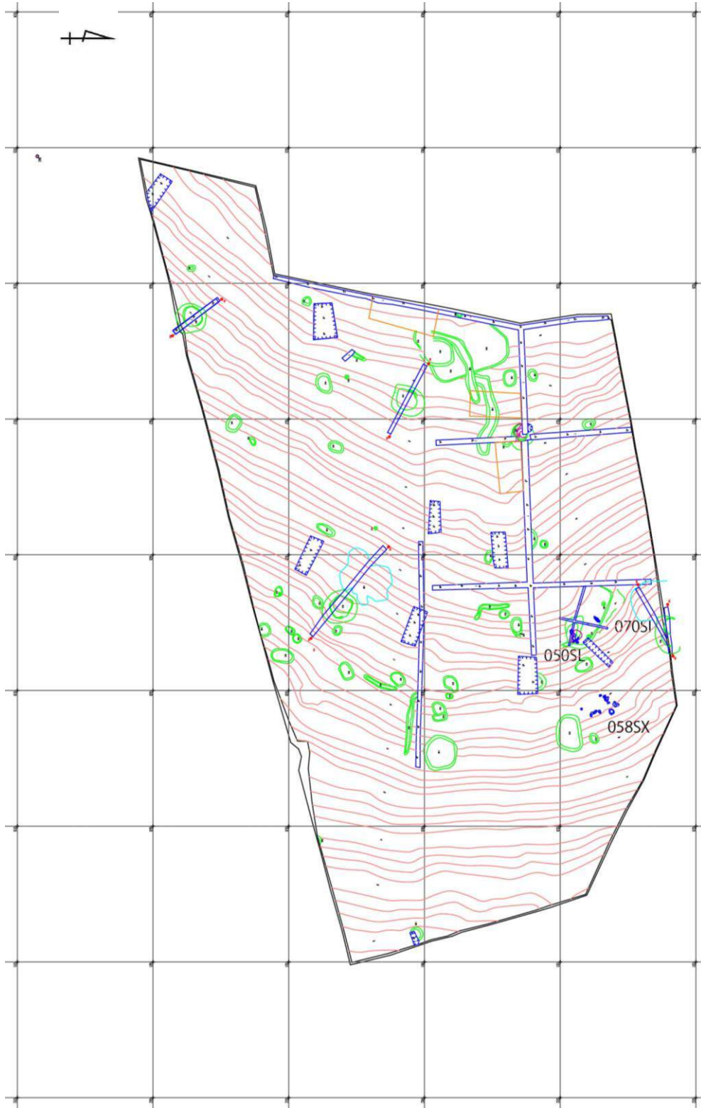
丸山遺跡遺構平面図 (1 : 400)
