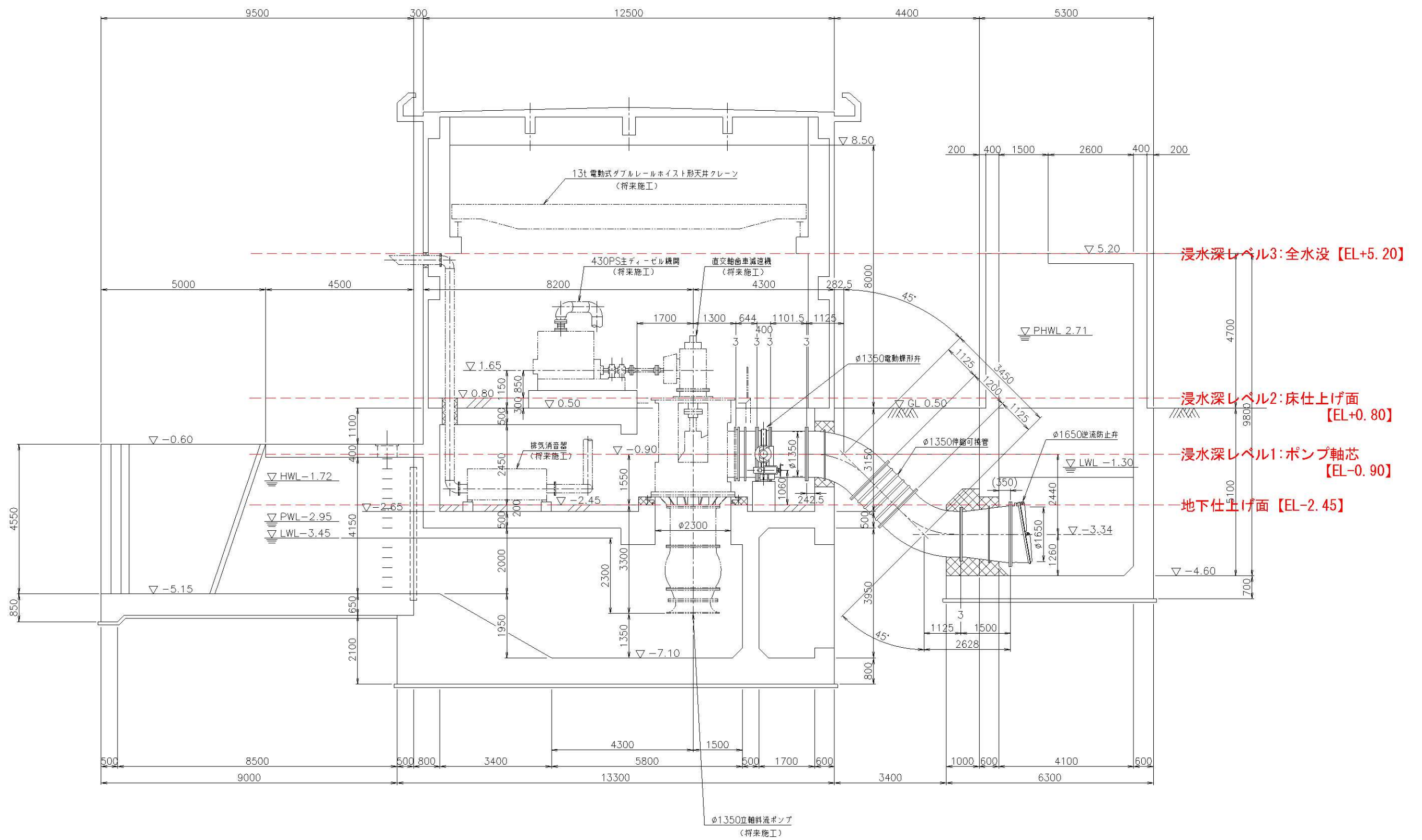
断面図
