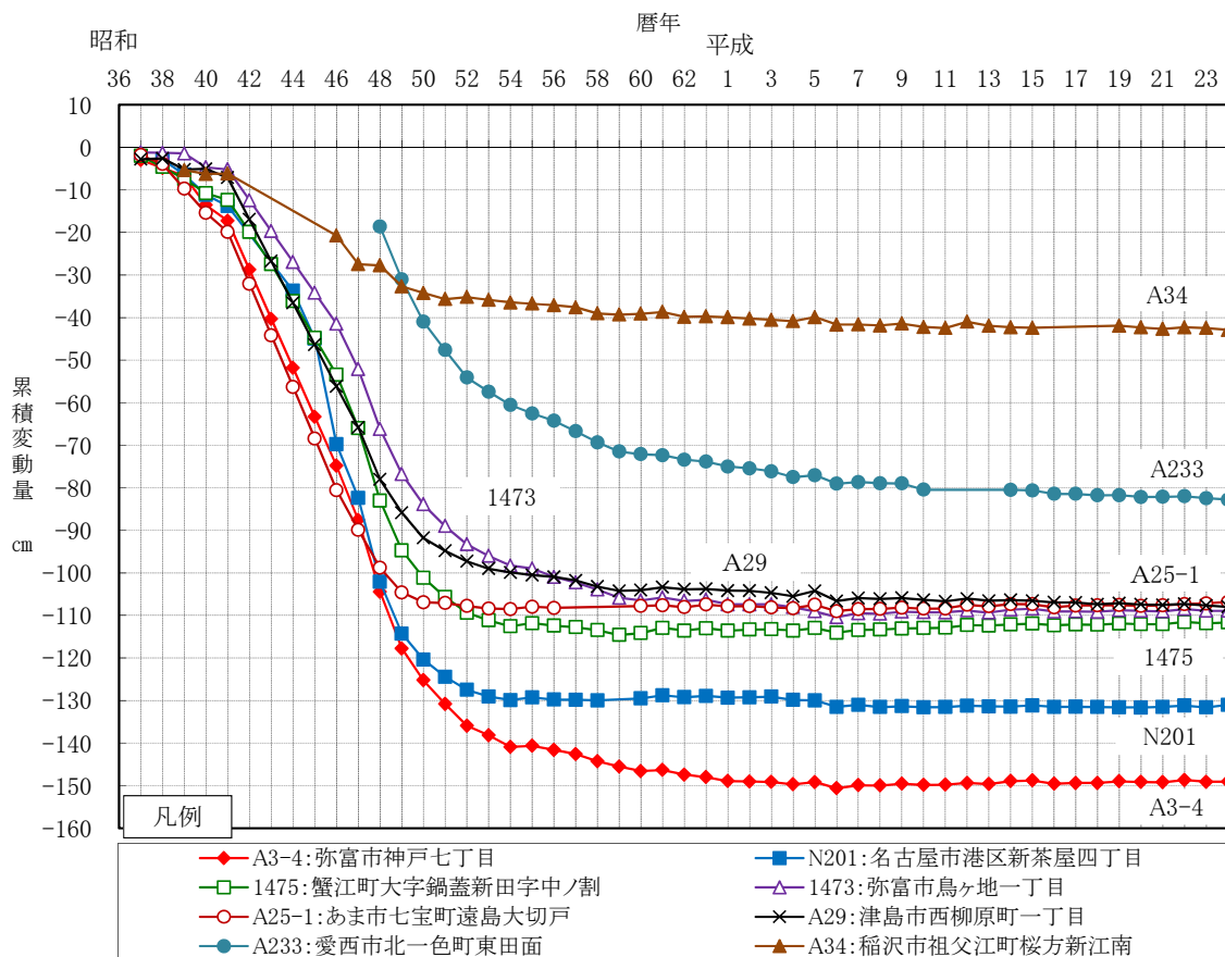
図1-3 主要な水準点の調査開始からの累積変動状況(尾張・名古屋市地域)
