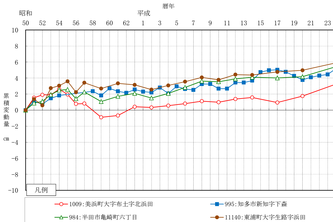
図 1-5 主要な水準点の累積変動状況（知多地域）
