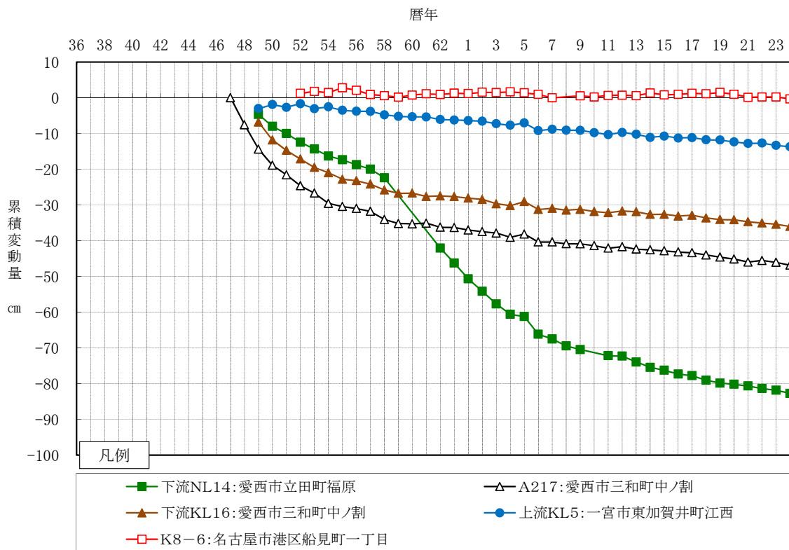
図1-2 最近5年間の累積沈下量の大きい水準点の変動状況(尾張・名古屋市地域)
