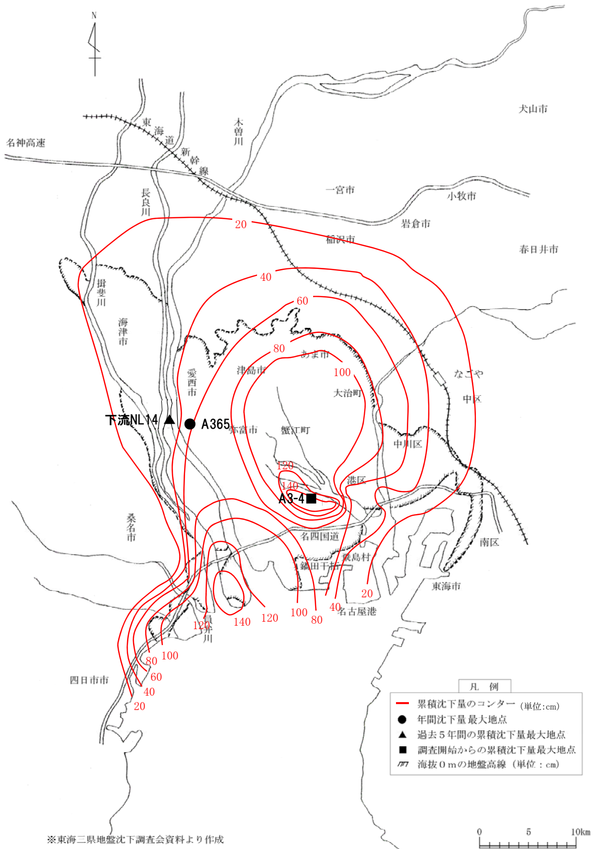
図1-4 累積沈下量のコンター図 (昭和36年~平成24年.尾張・名古屋市地域)
