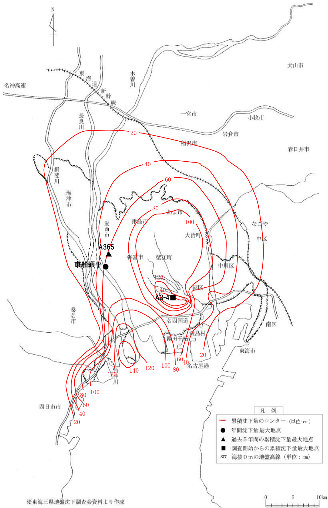
図1-4 累積沈下量のコンター図 (1961年～2020年:尾張・名古屋市地域)
