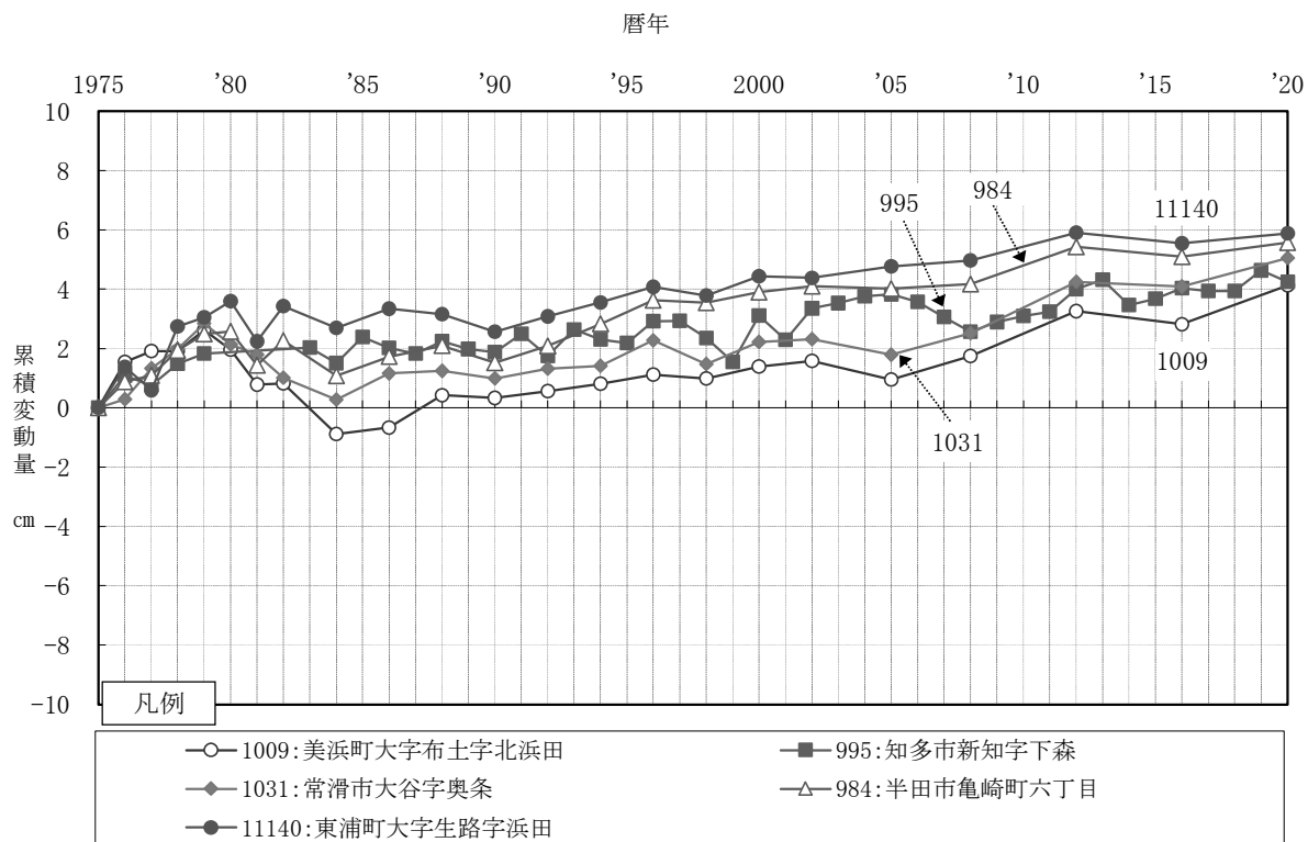
図1-5 主要な水準点の累積変動状況（知多地域）
