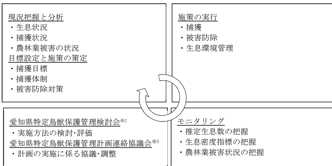
図 12 順応的管理
