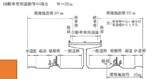
図 3.4 環境施設帯（自動車専用道路等の場合） 【参考】道路構造令の解説と運用，P171～，平成16年2月，（社）日本道路協会
