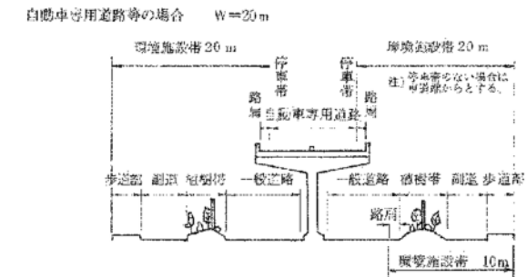
図 3.4 環境施設帯（自動車専用道路等の場合） 【参考】道路構造令の解説と運用，P171～，平成16年2月，（社）日本道路協会
