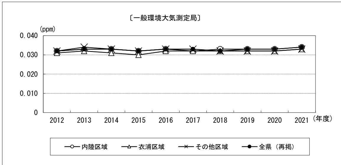
図1-7 一般環境大気測定局における光化学オキシダントの区域別年平均値の経年変化
