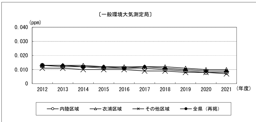
図1-4 一般環境大気測定局における二酸化窒素の区域別年平均値の経年変化
