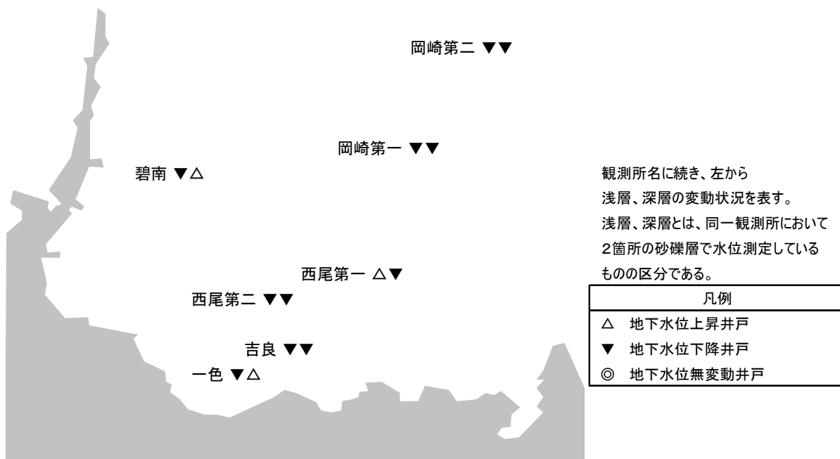
図2-7 西三河観測井の地下水位変動状況(平成24年と25年の平均地下水位比較)
