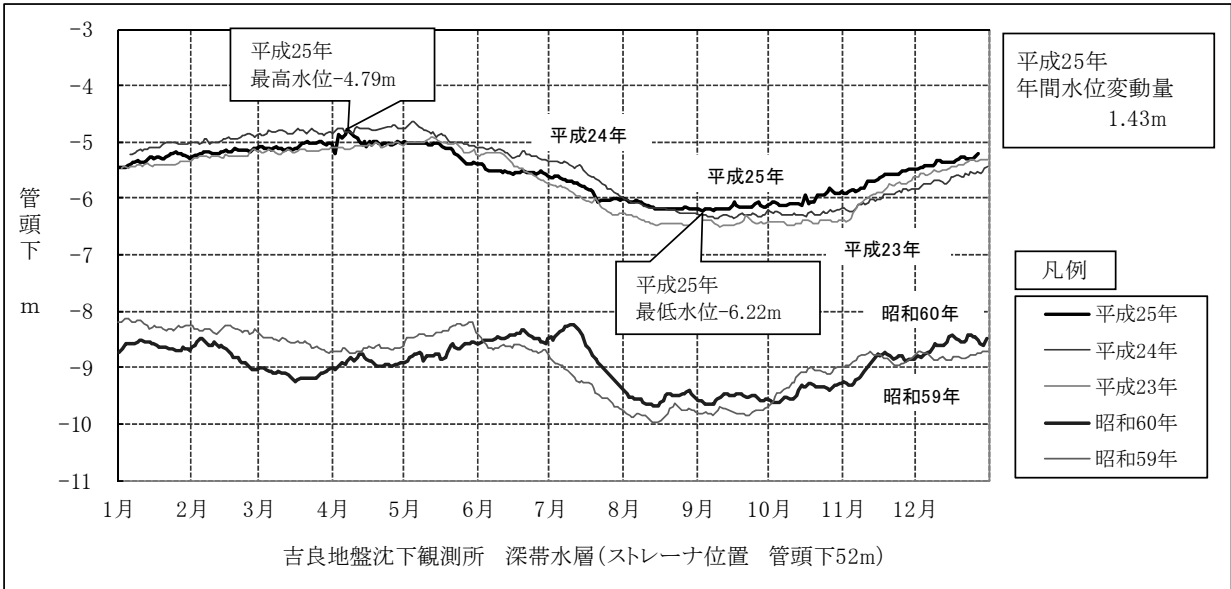
図 2 - 13 年別地下水位変動状況 (吉良地盤沈下観測所)
