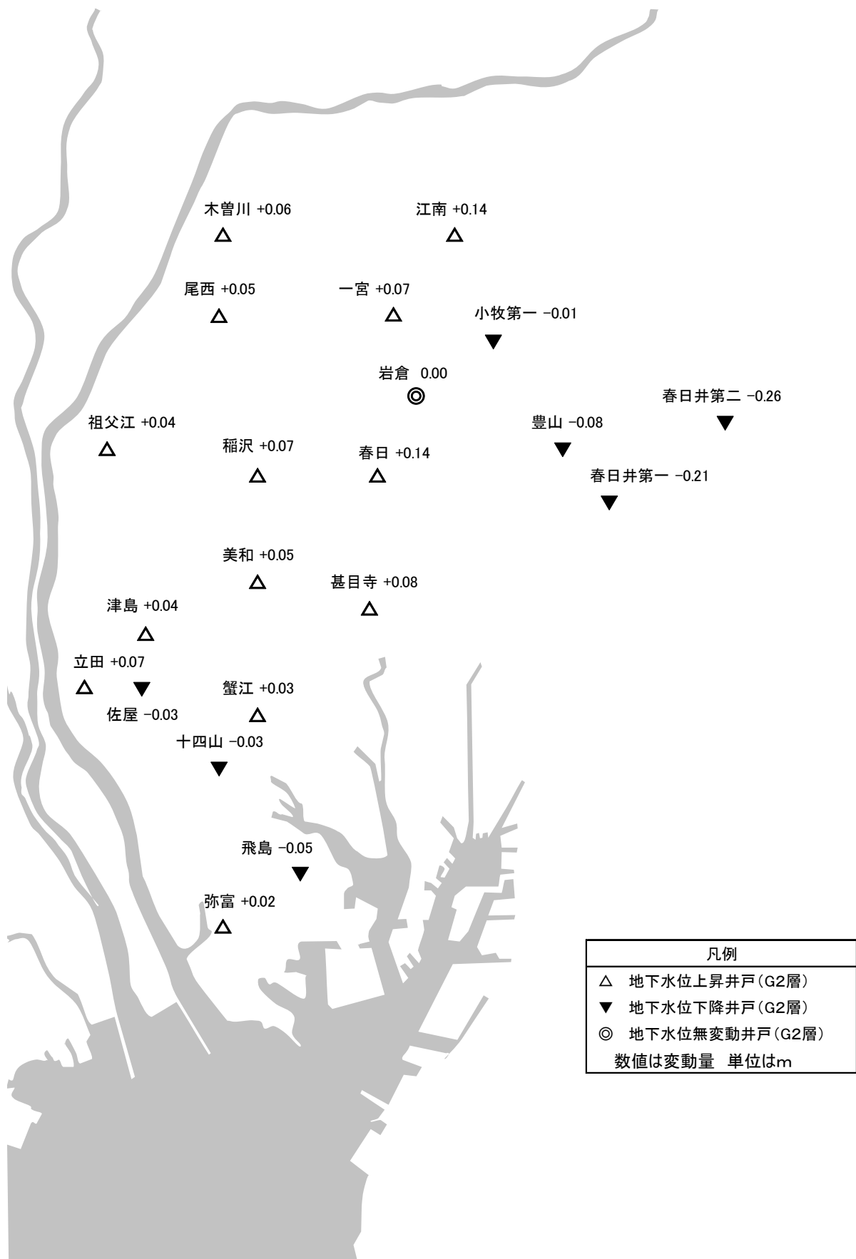
図 2 - 4 観測井 G 2 層の地下水位変動状況 (21 井) (平成 24 年と 25 年の平均地下水位比較)
