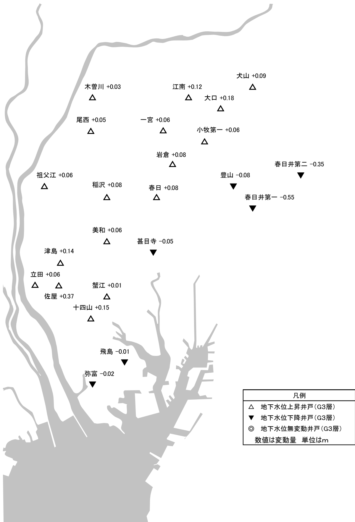
図 2 - 5 観測井 G 3 層の地下水位変動状況 (23 井) (平成 24 年と 25 年の平均地下水位比較)
