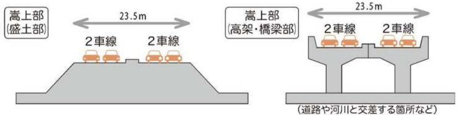
【横断図】
