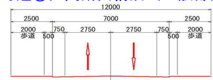
町道③区間断面構成（一般部）
