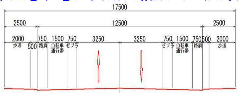
県道①、②区間断面構成（一般部）
