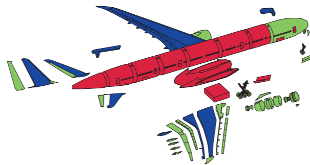
ボーイング 777X 製造分担図（製造割合21%）
