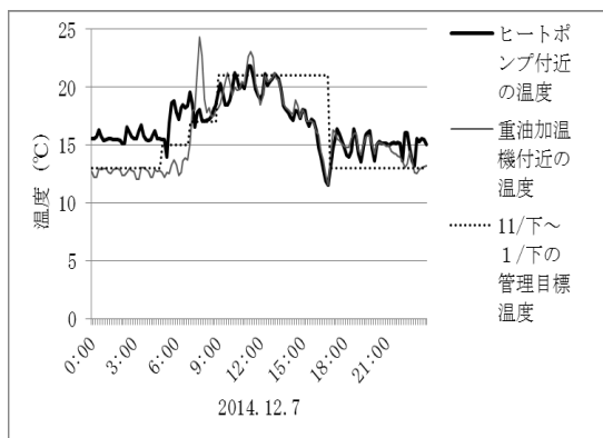
図1 併用区におけるヒートポンプ付近、重油加温機付近の温度推移
