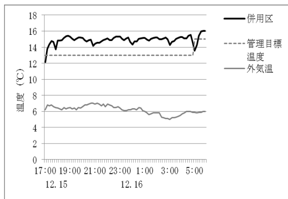
図2 併用区の夜間（17時～6時）までの施設内の温度推移
