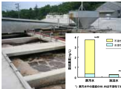
豚舎浄化槽による亜鉛除去効果を解明
