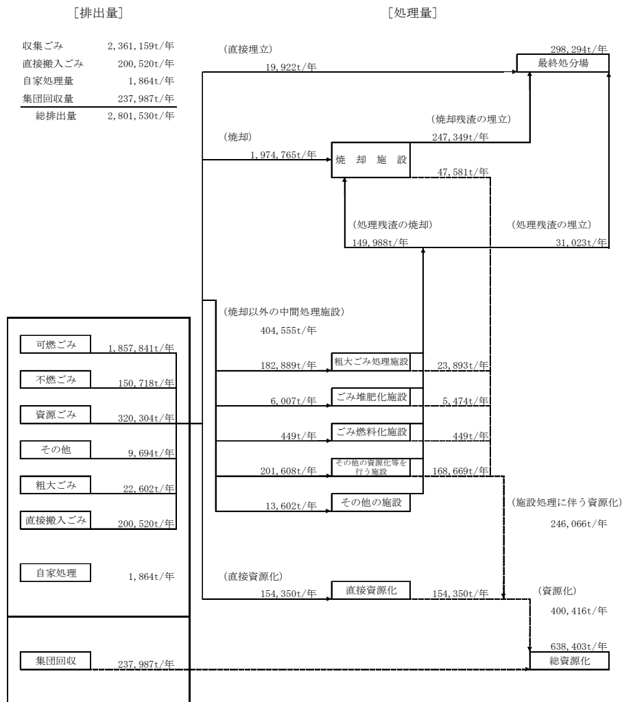
図 3 ごみ処理の流れ (平成 20 年度)
