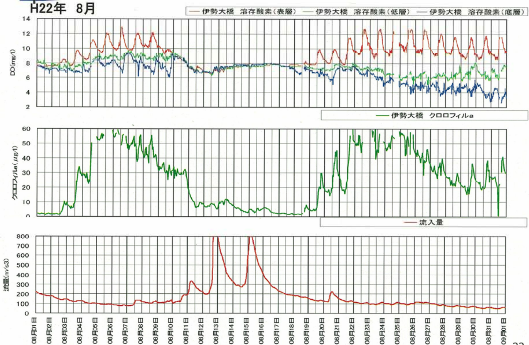
図10-1 河口堰上流(伊勢大橋)のDOとクロロフィルa・流量
