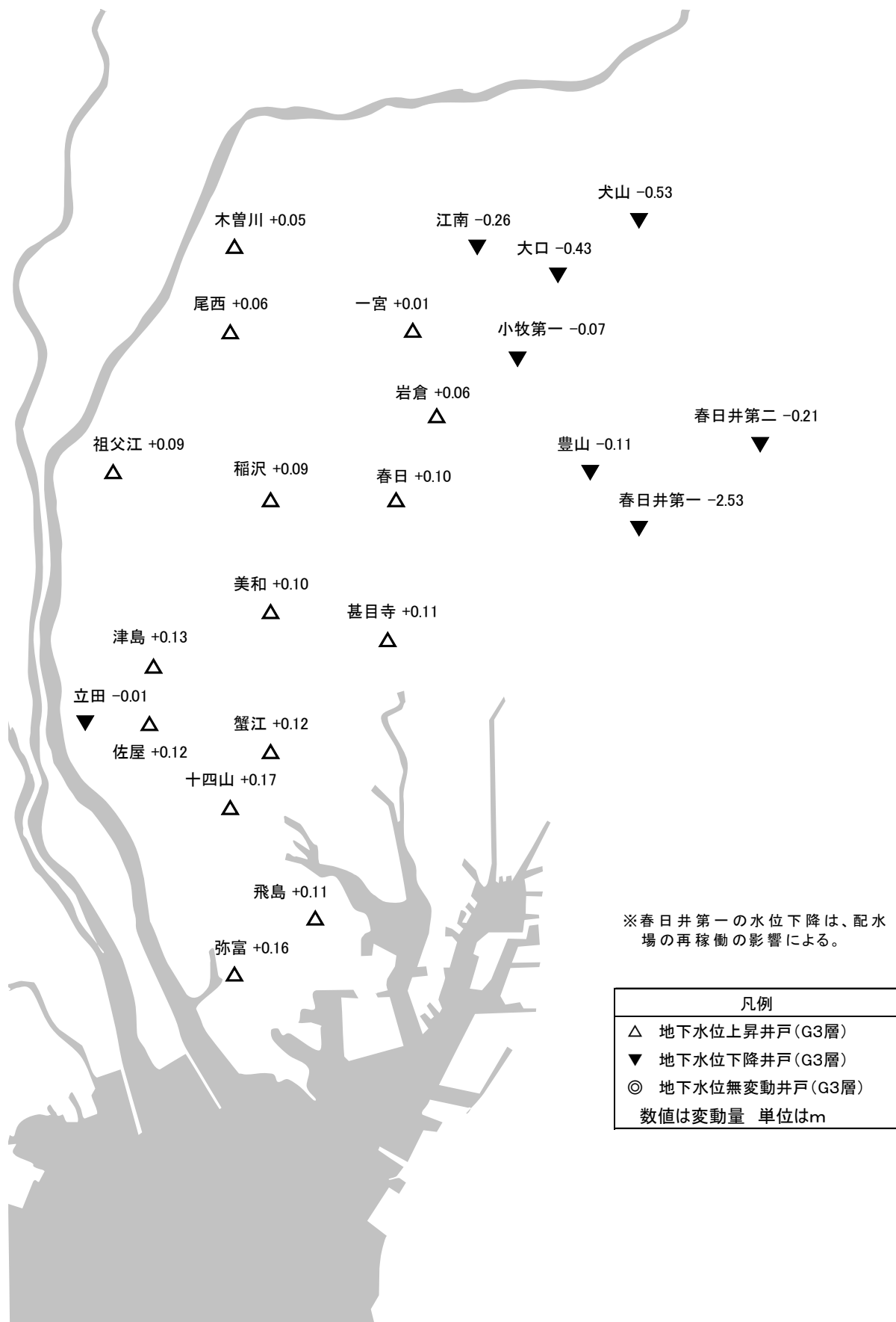
図 2 - 5 観測井 G 3 層の地下水位変動状況 (23 井) (平成 28 年と 29 年の平均地下水位比較)
