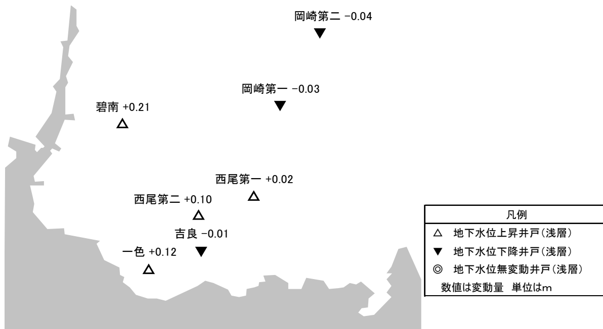
図 2 - 8 西三河浅層の地下水位変動状況 (7井) (平成 28 年と 29 年の平均地下水位比較)
