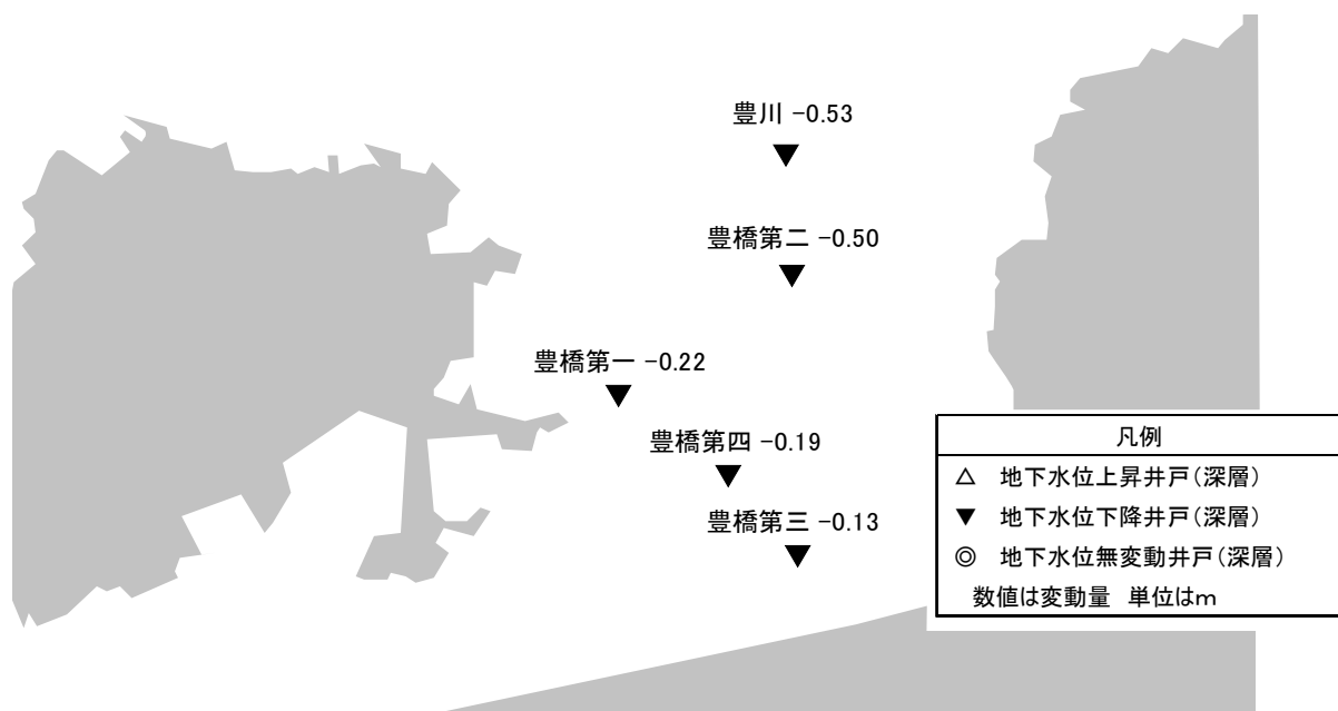
図 2 - 13 東三河深層の地下水位変動状況 (5井) (平成 28 年と 29 年の平均地下水位比較)
