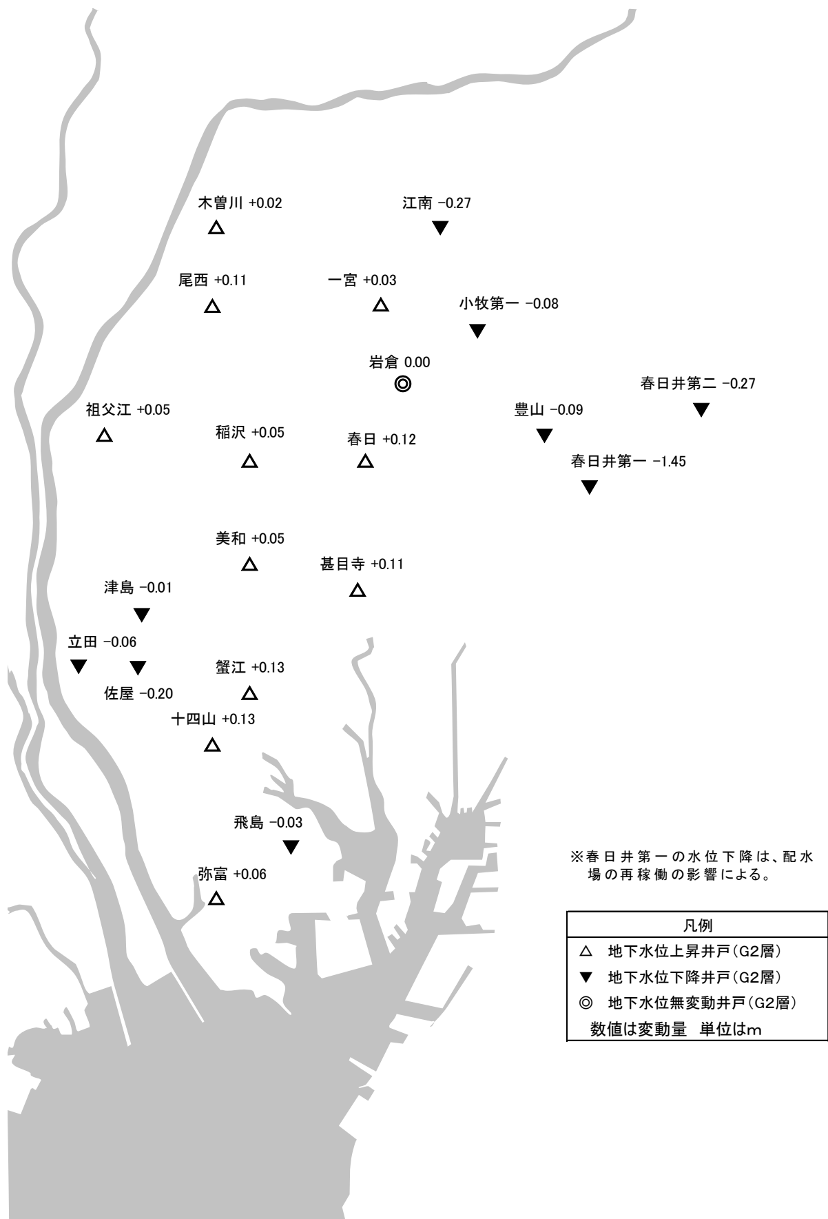
図2-4 観測井G2層の地下水位変動状況(21井) (平成28年と29年の平均地下水位比較)
