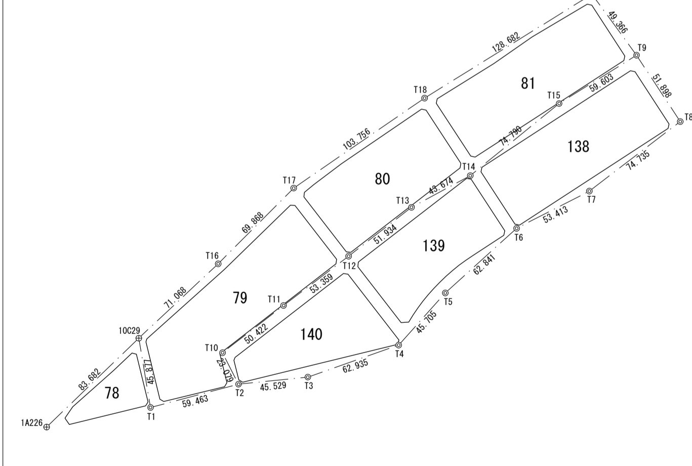
基準点・多角点配置図 縮尺 1 : 2500
