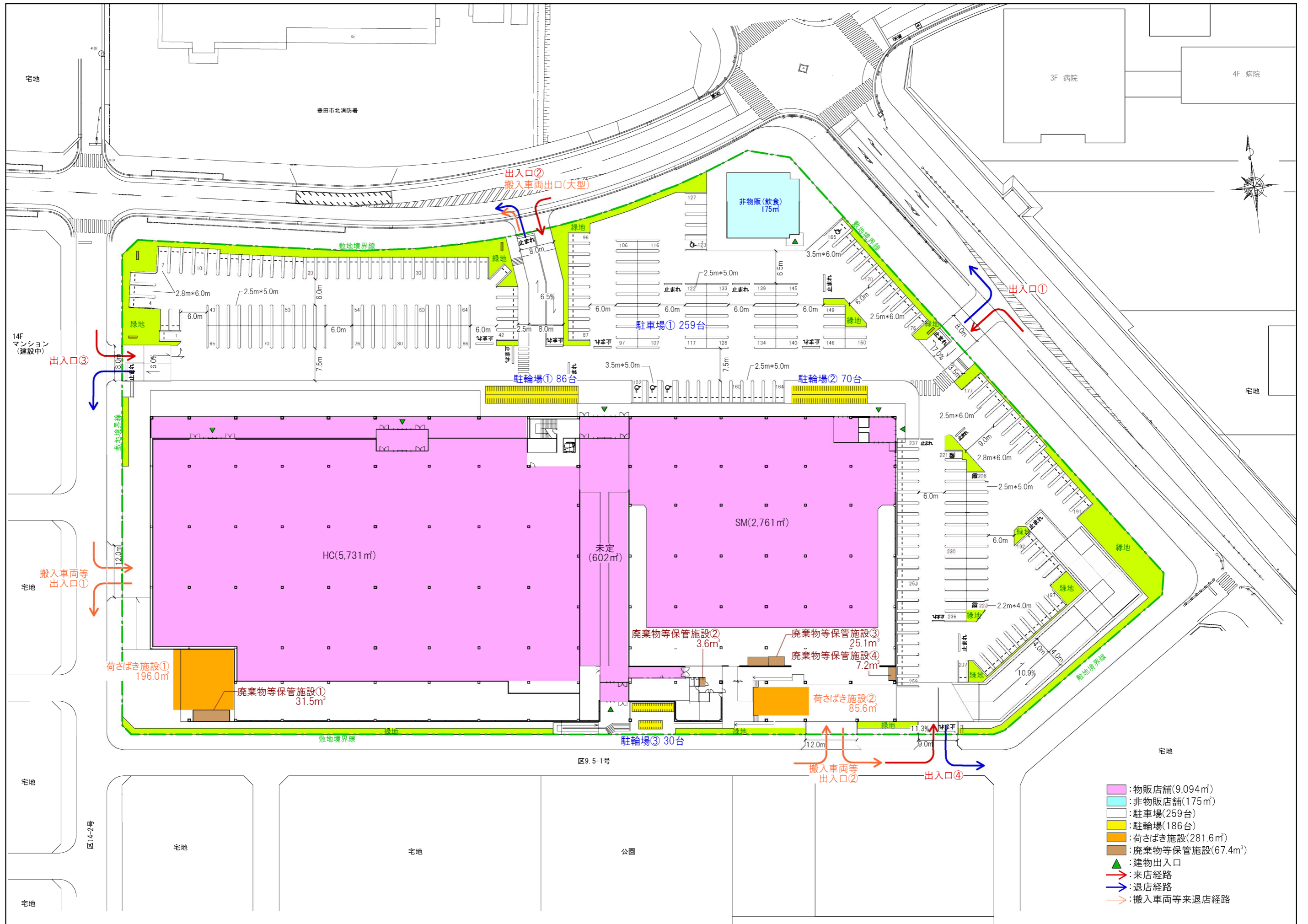
別添図面4 配置図兼1階平面図(1/800)
