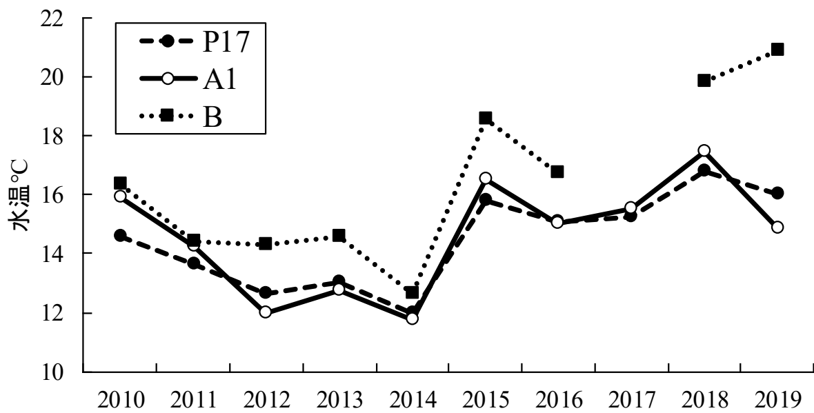
図2 調査点の底層水温の推移 (12月下旬)
