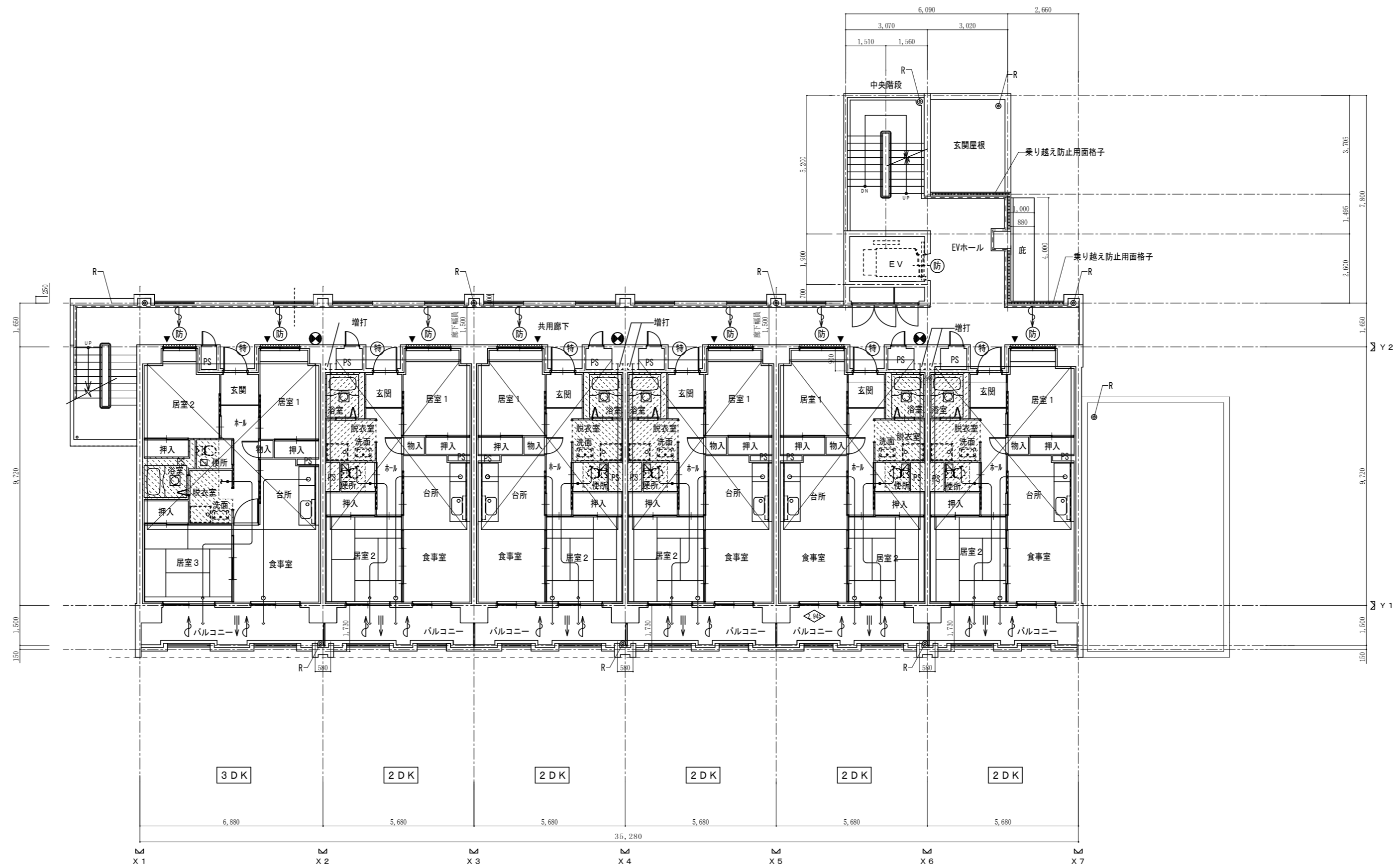
2階平面図 S=1/100 (東棟)
