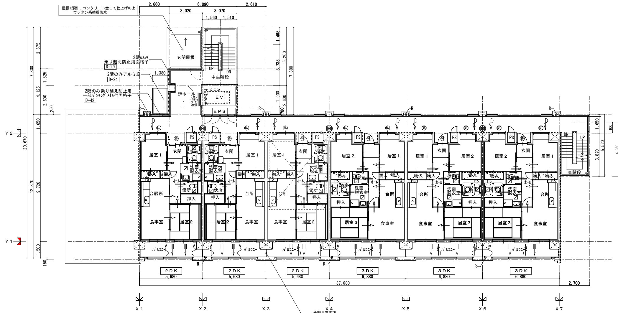
2~7階 平面図 S=A1: 1/100・A3: 1/200
