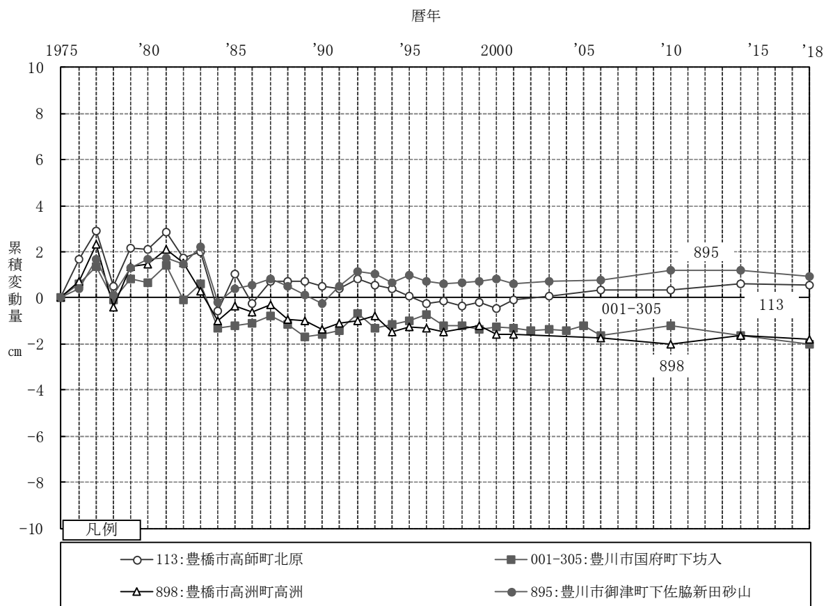
資料図 7－1 主要な水準点の調査開始からの累積変動状況（東三河地域）
