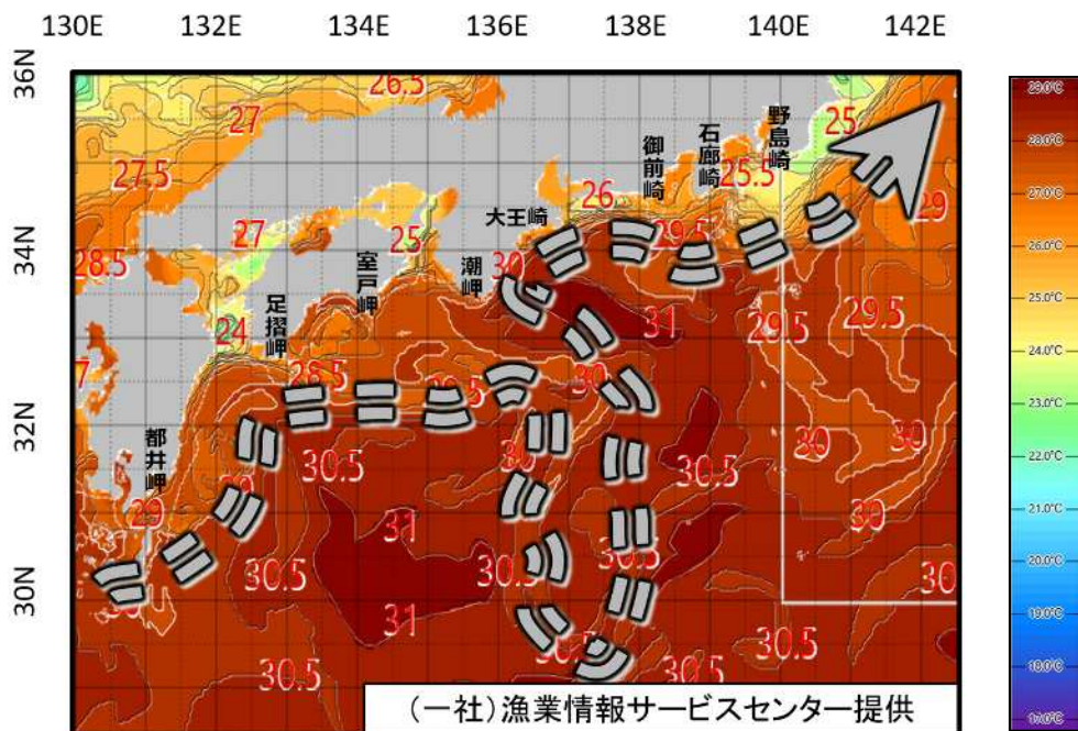
8月18日の水温分布と黒潮流路（広域図）
