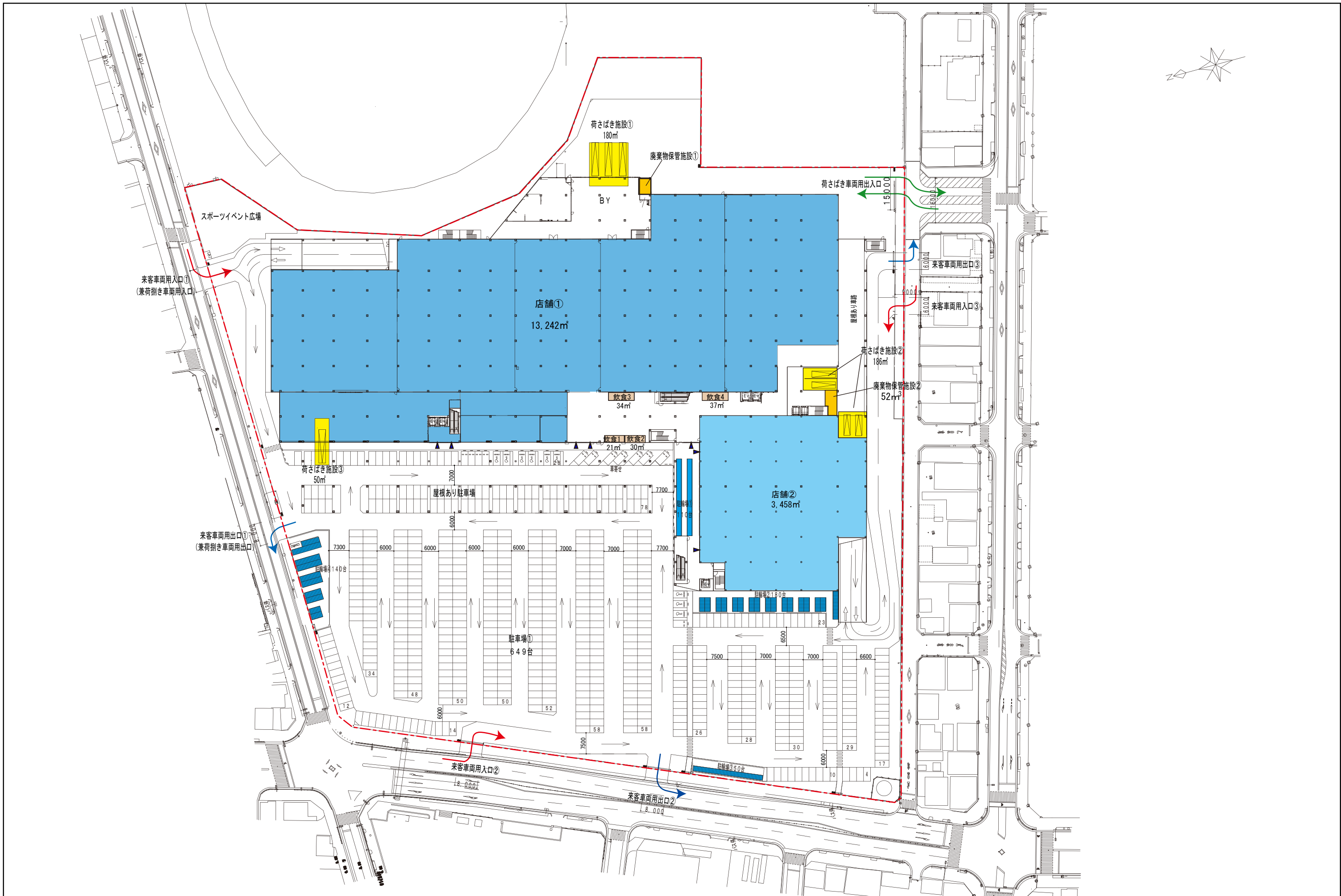
図面3 建物配置図兼1階平面図 (S=1/1,200)
