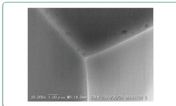
図2 CMP加工による三角錐刃先
