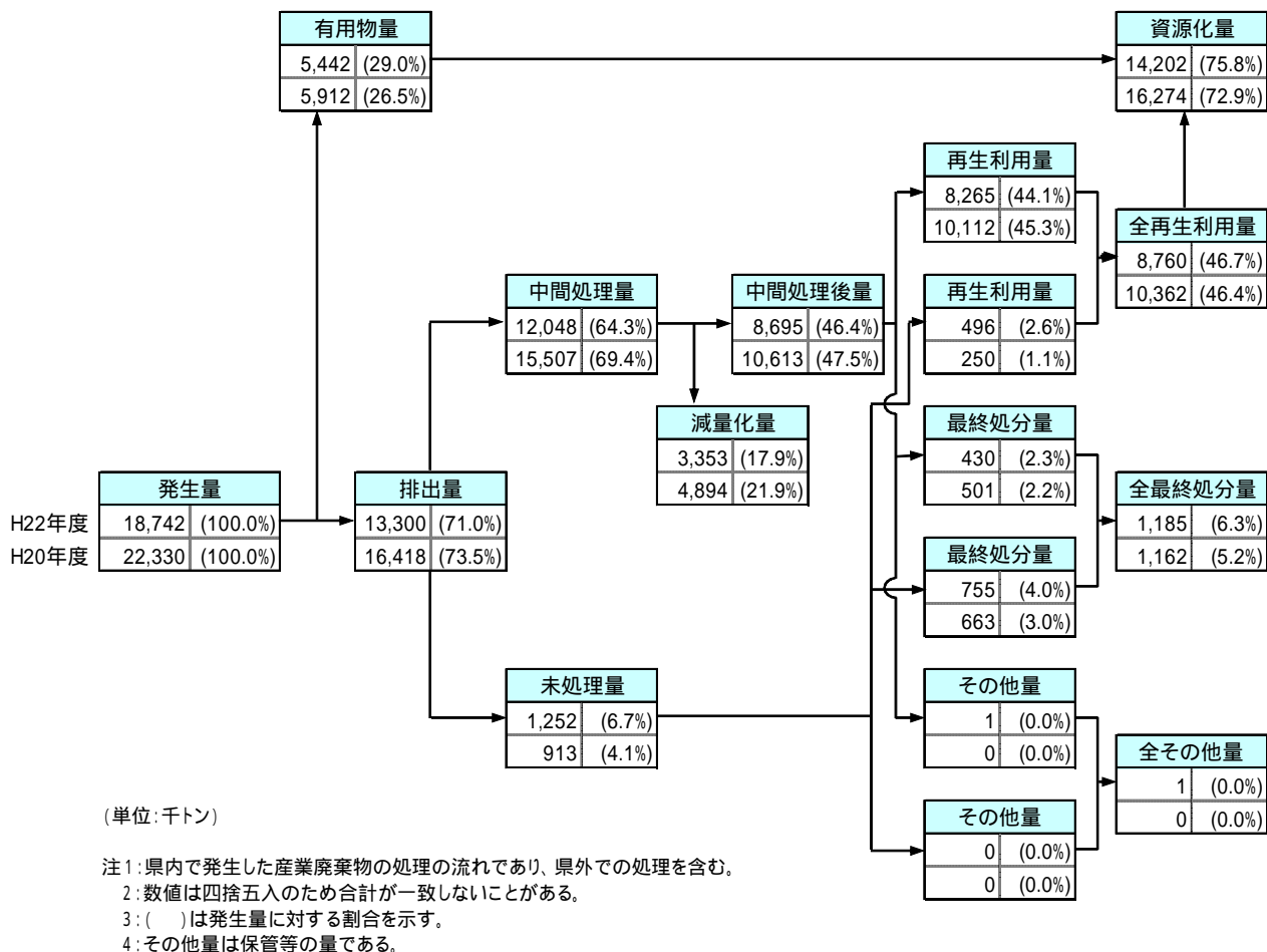
図 1 -(1)-6 産業廃棄物の処理の流れ
