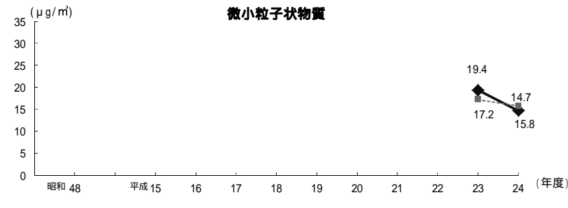
図1-3 全県年平均値の経年変化
