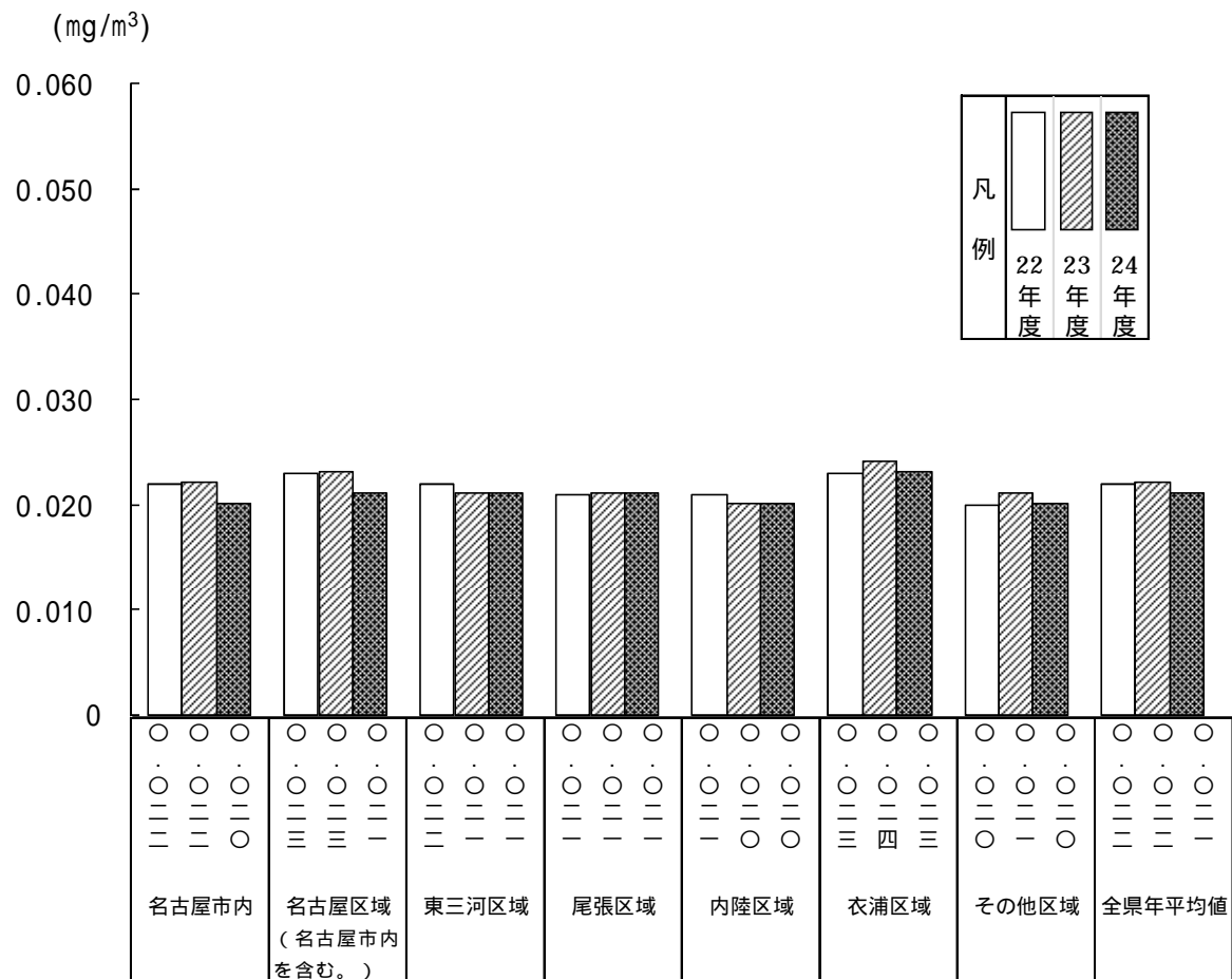
図1-9 浮遊粒子状物質の区域別年平均値の経年変化（一般環境大気測定局）
