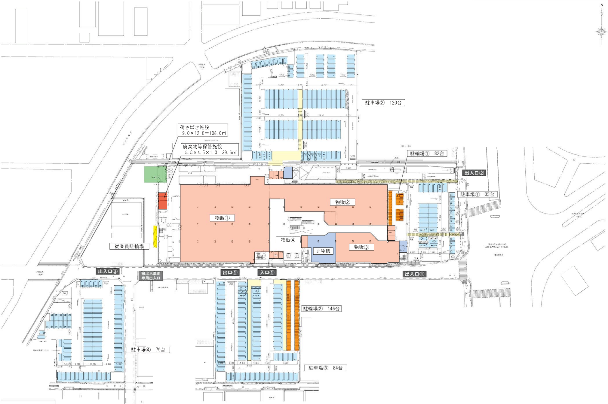
図面3 建物配置図及び1階平面図
