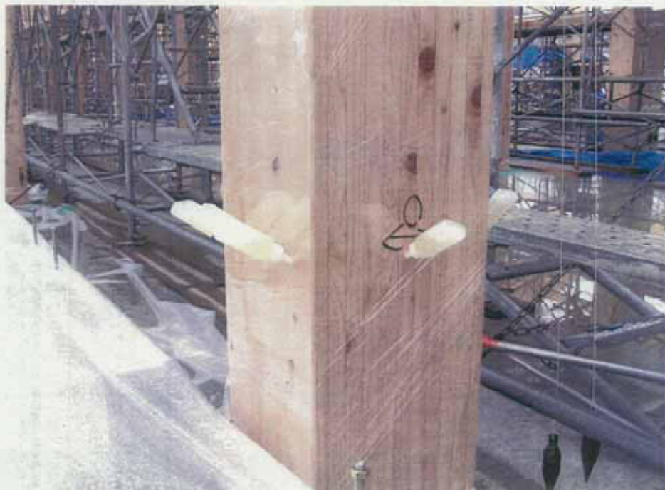
集成材樹脂注入(柱脚部)
