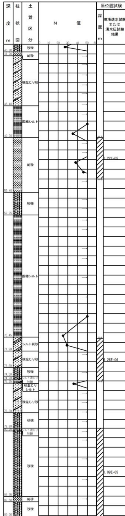
ボーリング柱状図 (No. 3) 1/1
