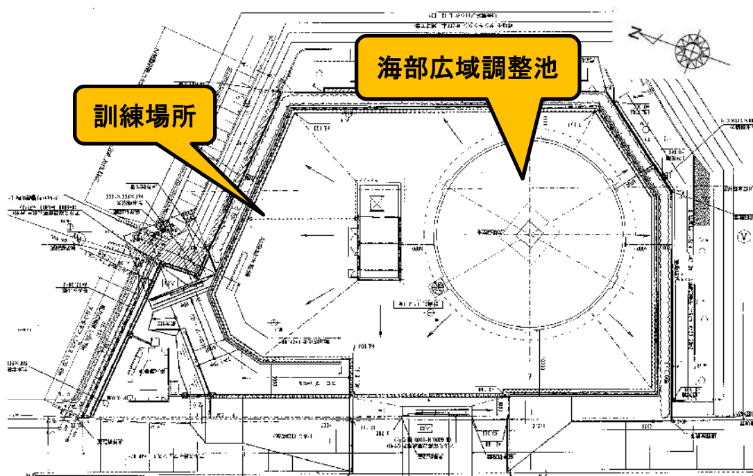
平面図
