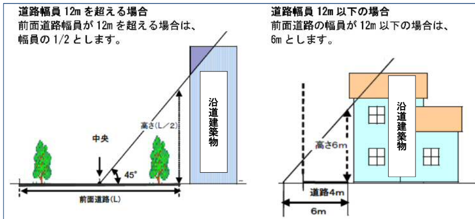
図-2 倒壊時に道路の半分を閉塞するおそれのある建築物
