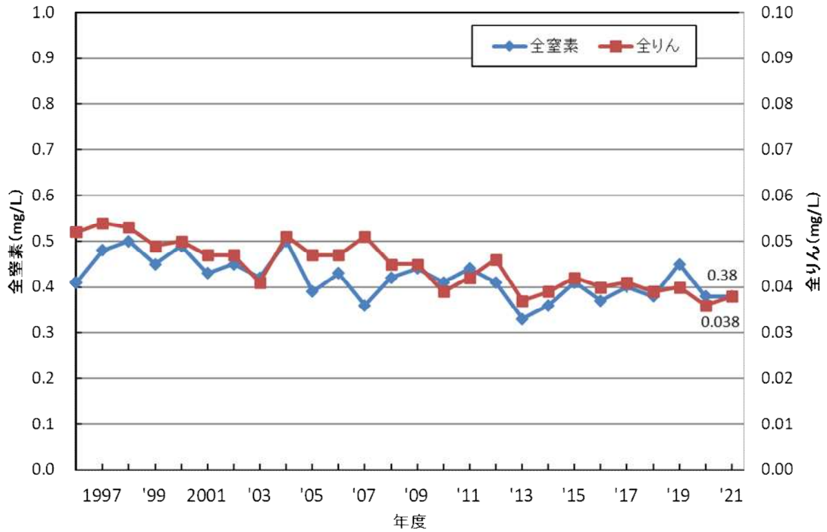
(参考8) 海域における全窒素及び全りん濃度推移 (年間平均値)
