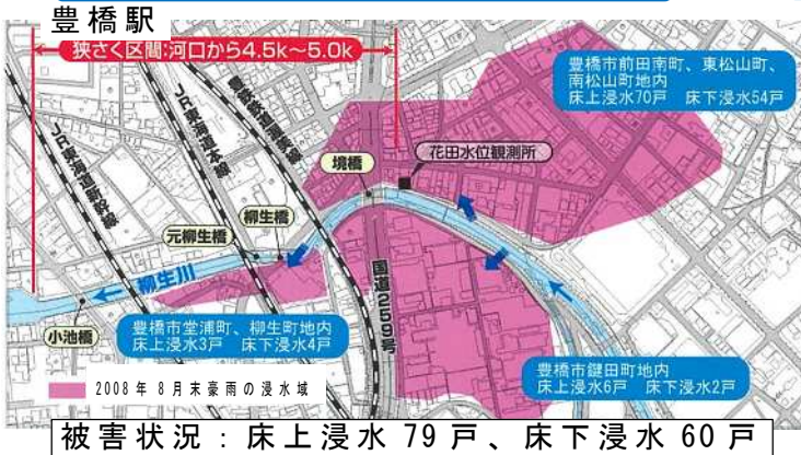
地下河川の整備効果
