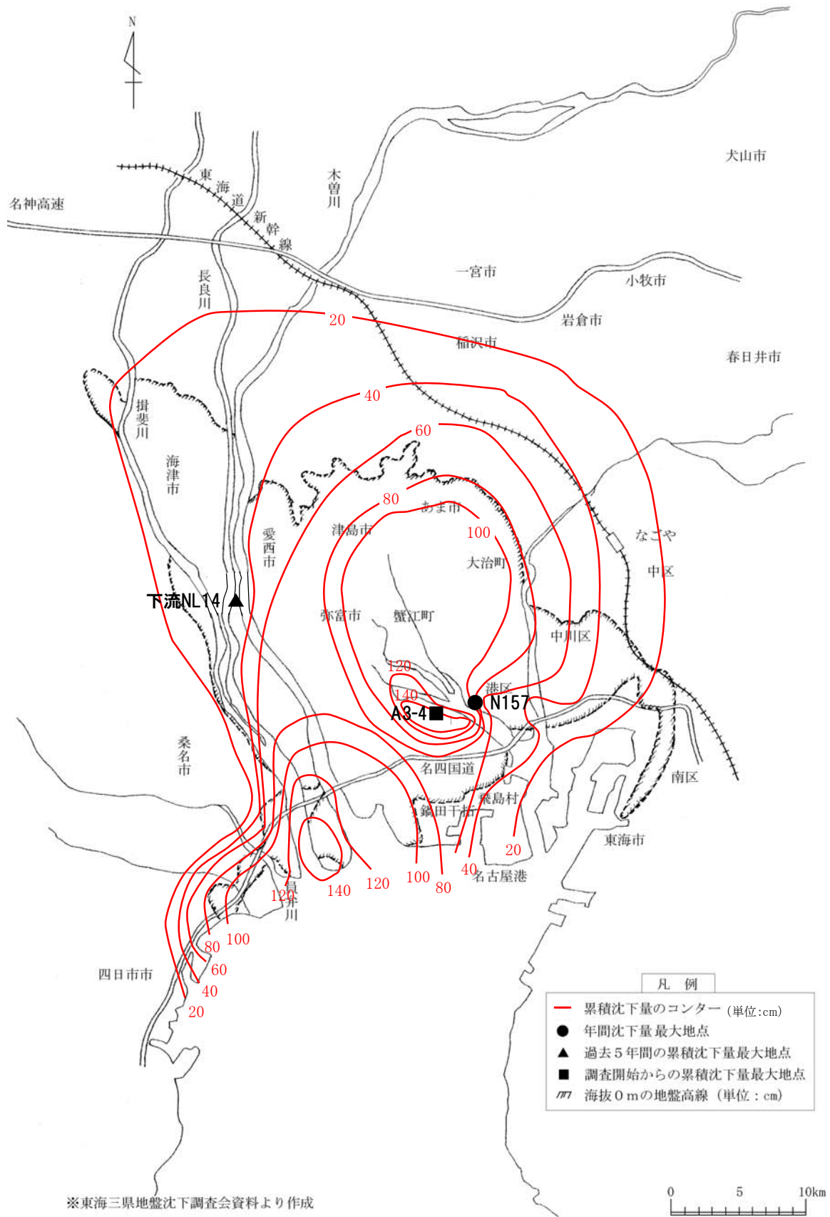
図1-4 累積沈下量のコンター図 (昭和36年~平成25年、尾張・名古屋市地域)
