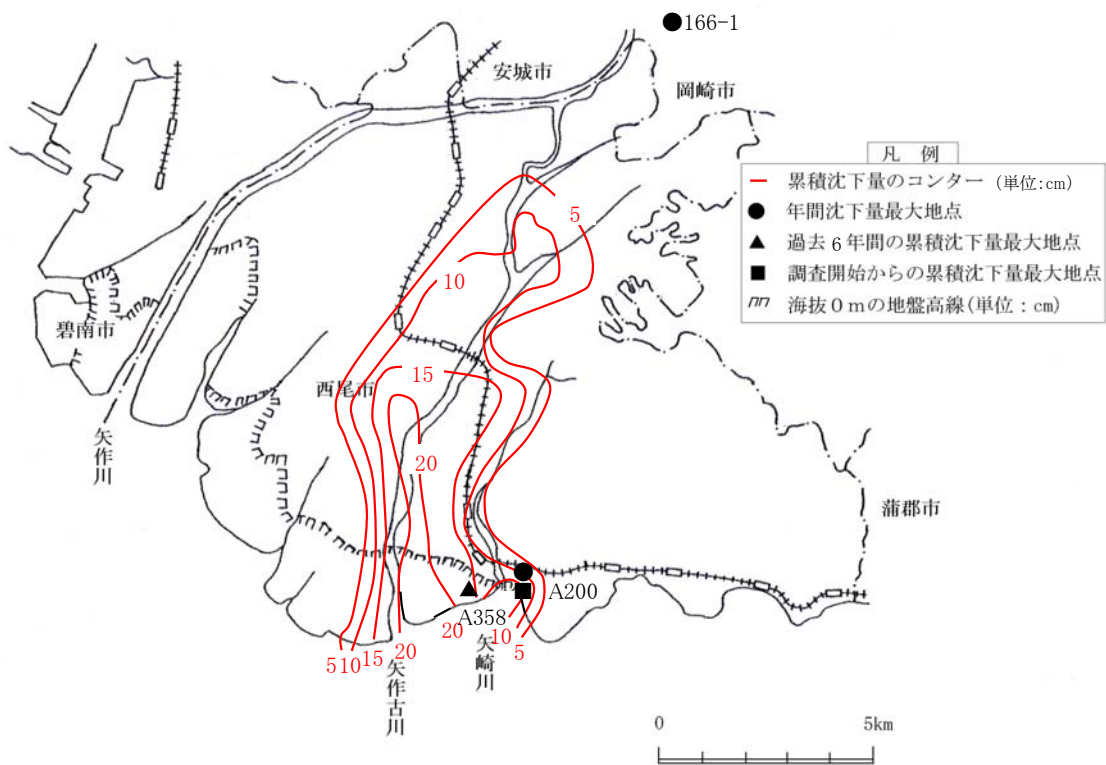
図 1 - 7 累積沈下量のコンター図（昭和 50 年～平成 25 年、西三河地域）
