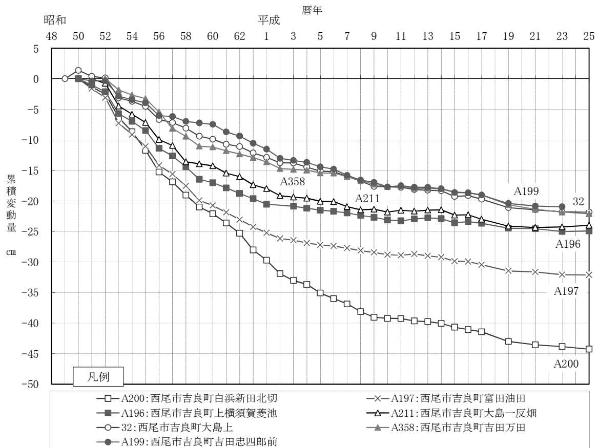
図 1 - 6 主要な水準点の累積変動状況（西三河地域）
