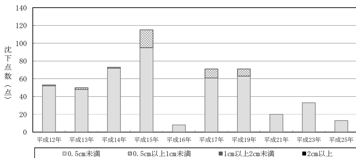
図 1 - 5 沈下を示した水準点の数（西三河地域）
