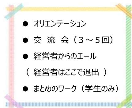
〔プログラム〕
