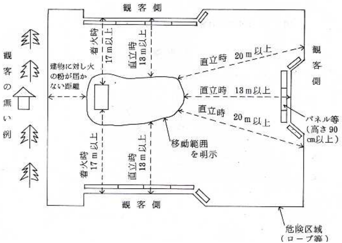
手筒花火の消費図 (薬量2, 400g)
