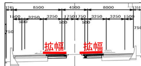
【道路断面図(4車線化部)】
