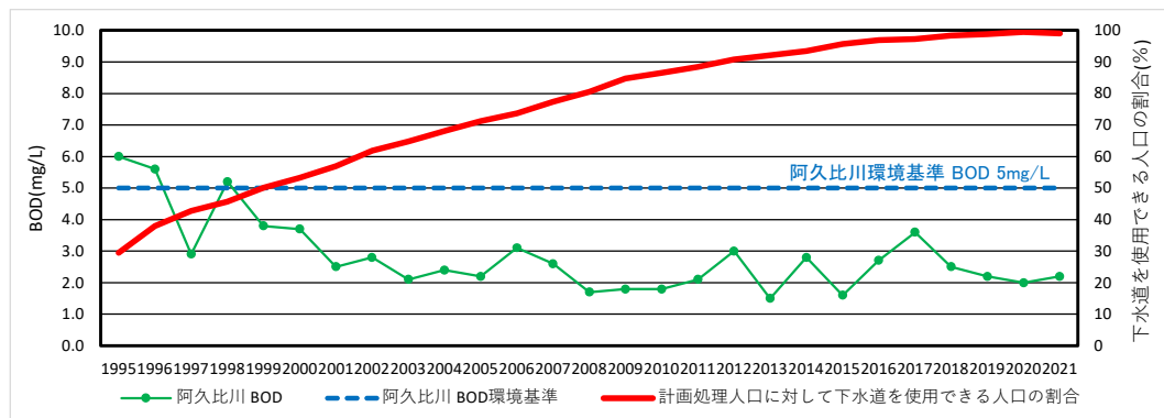
衣浦西部流域下水道計画区域内における河川水質 (BOD) の経年変化
