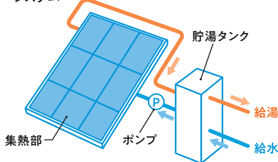
ソーラーシステム
