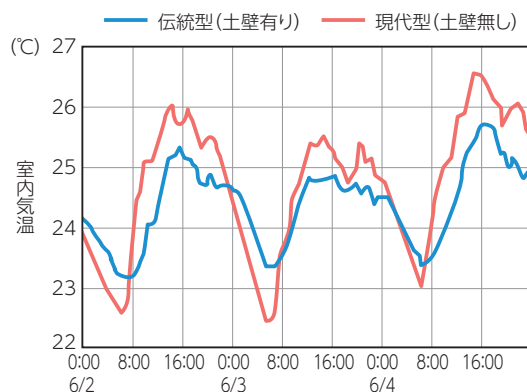
土壁と新材の温熱環境シミュレーション (中間季における室内平均気温の変動)
