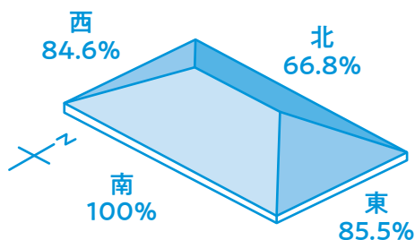
設置方位による発電量の割合 (屋根傾斜角30°)
