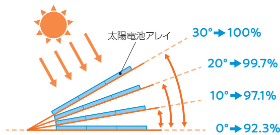
傾斜角による発電量の割合 (真南設置)
