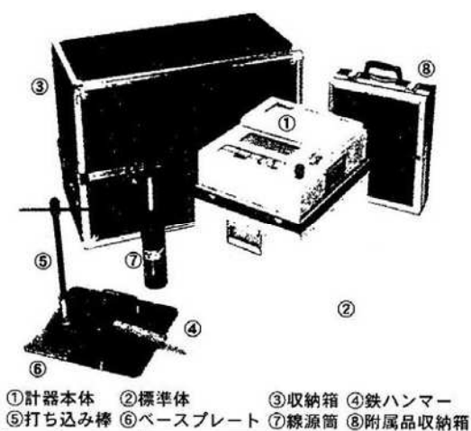
図-4 計器の構成例 (透過型)
