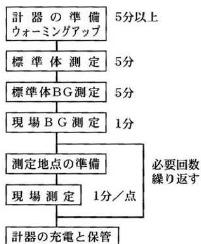
図-5 測定の手順の例
