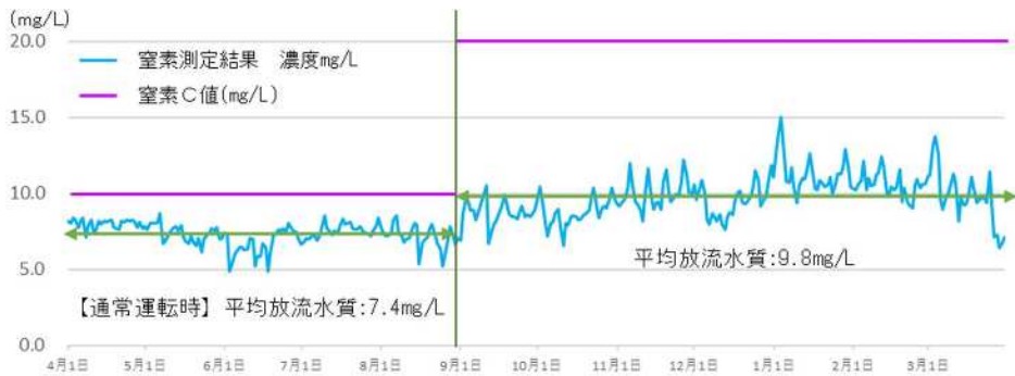
図1 矢作川浄化センターにおける社会実験(2023 年9月から 2024 年3月まで)による放流水の窒素濃度
