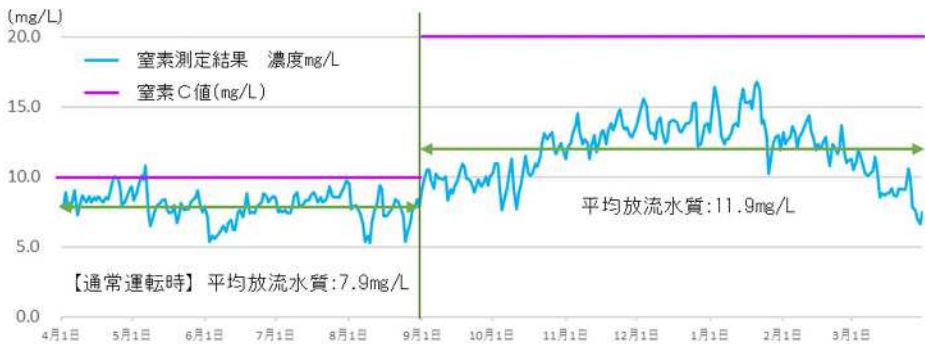
図2 豊川浄化センターにおける社会実験(2023 年9月から 2024 年3月まで)による放流水の窒素濃度
