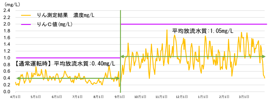
図4 豊川浄化センターにおける社会実験(2023 年9月から 2024 年3月まで)による放流水のリン濃度
