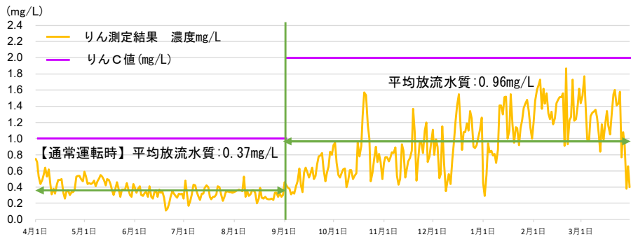
図3 矢作川浄化センターにおける社会実験(2023 年9月から 2024 年3月まで)による放流水のリン濃度
