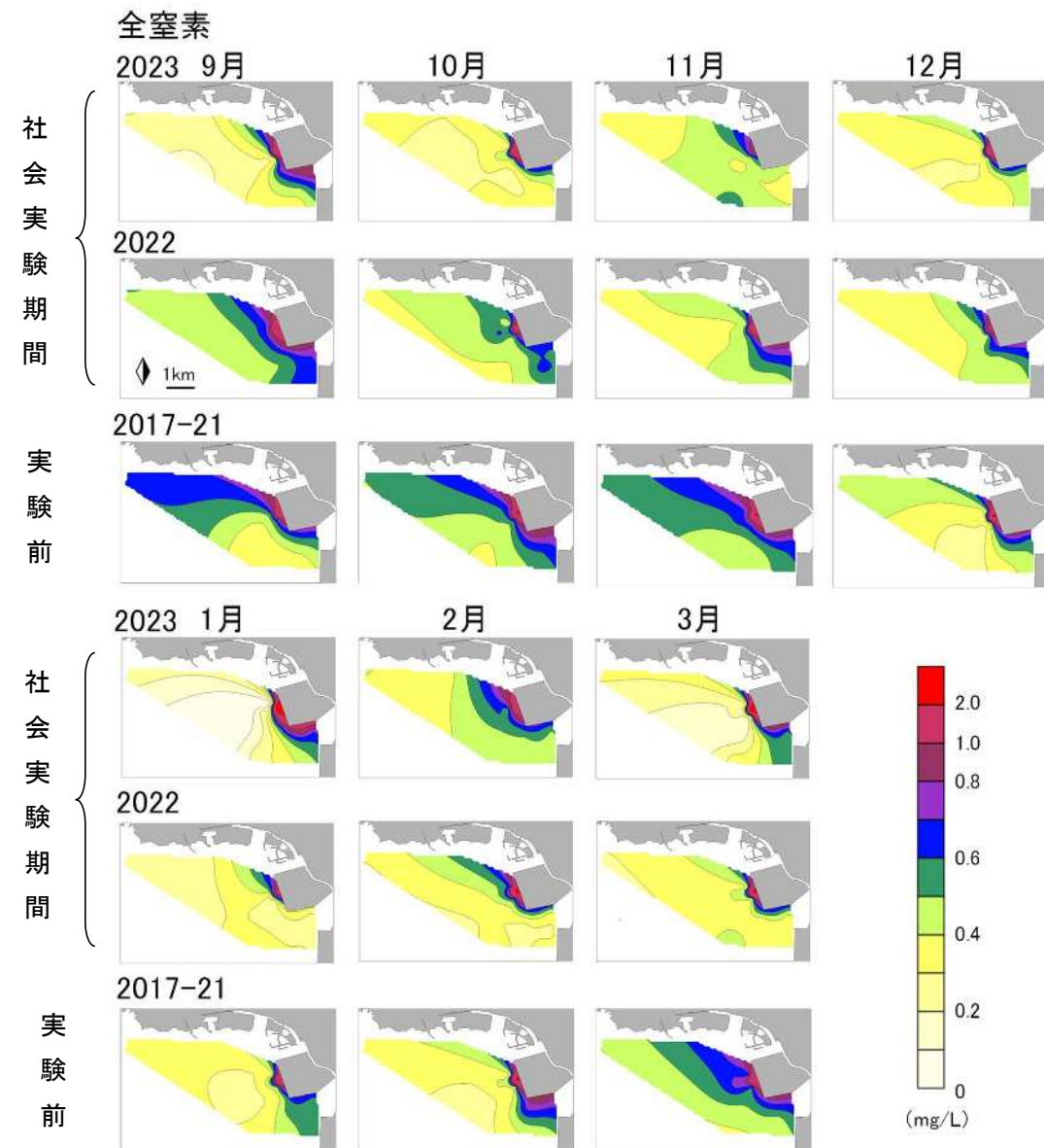
図 11 2023 年度、2022 年度及び社会実験前の過去 5 か年平均における豊川地区の全窒素濃度分布
