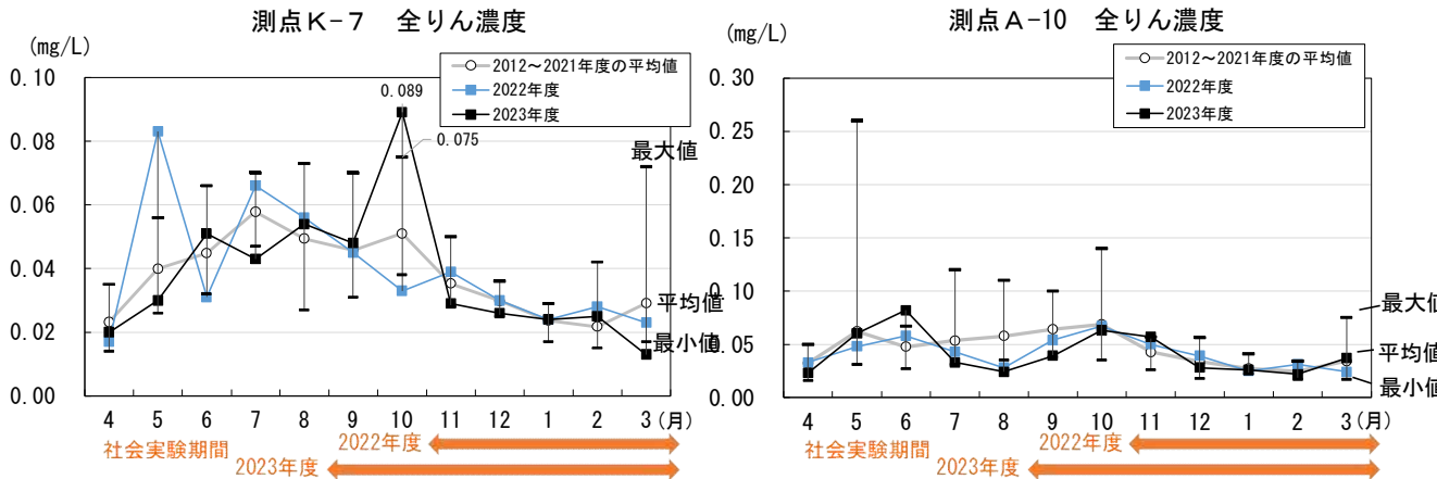
図 7 2022、2023 年度の測点 K-7・A-10 の月別全リン濃度及び過去 10 年間の平均値と最大値・最小値
