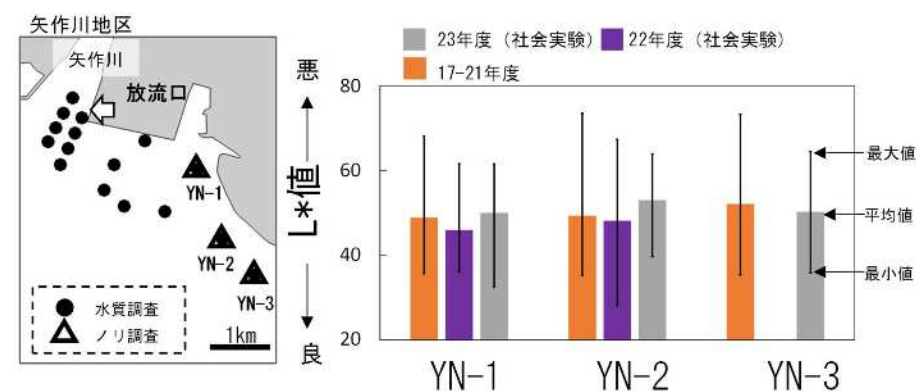
図 13 矢作川地区におけるノリ葉体の平均 L*値及び最大値と最小値
