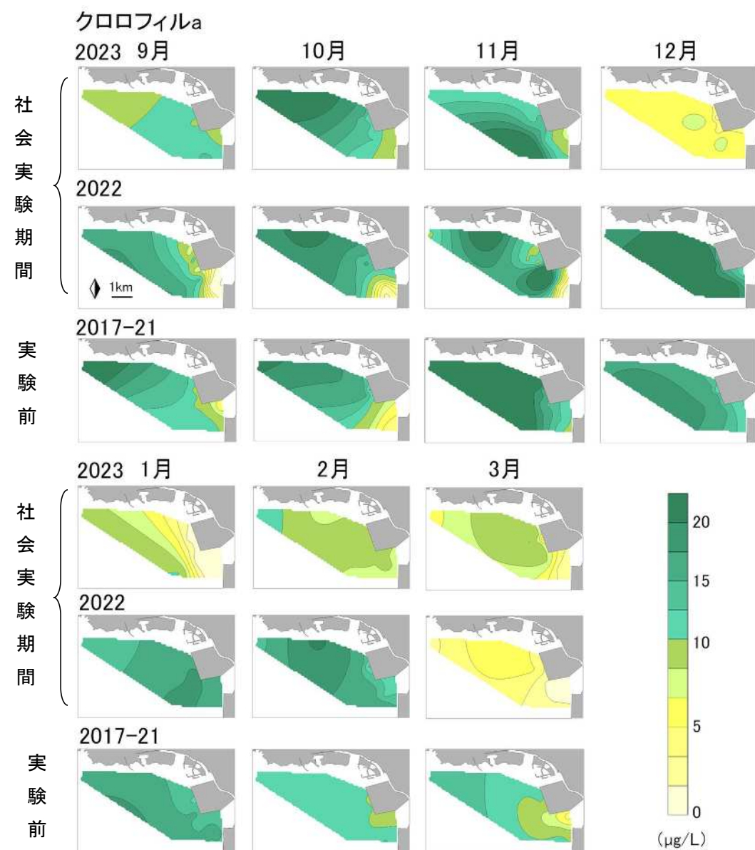
図 16 2023 年、2022 年及び社会実験前の過去 5 か年平均における豊川地区のクロロフィル a 濃度分布
