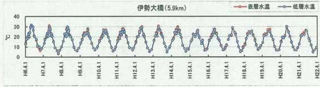
図 5.4.4(1) 水温経月変化 (H6年4月-H22年3月)
