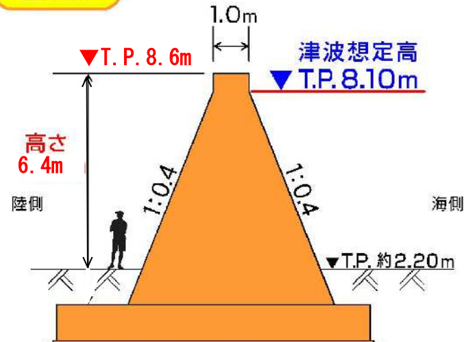
断面図
