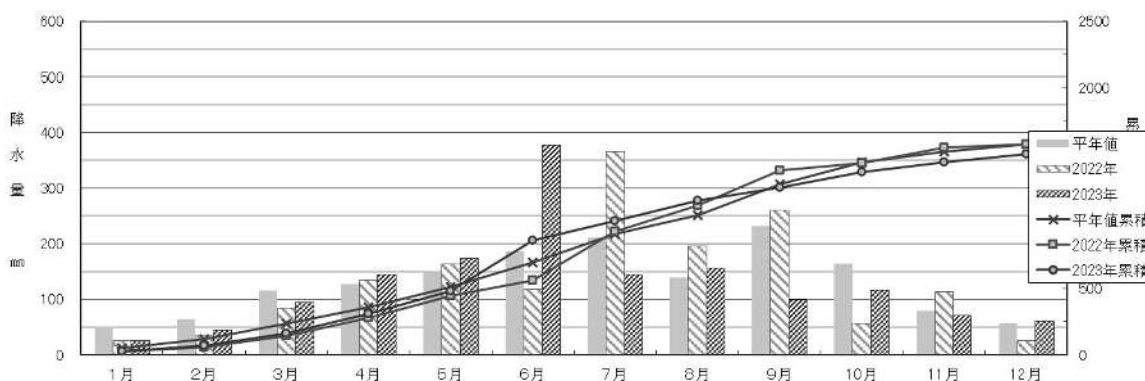
資料図6－1 名古屋地方気象台における月別降水量と累積降水量
